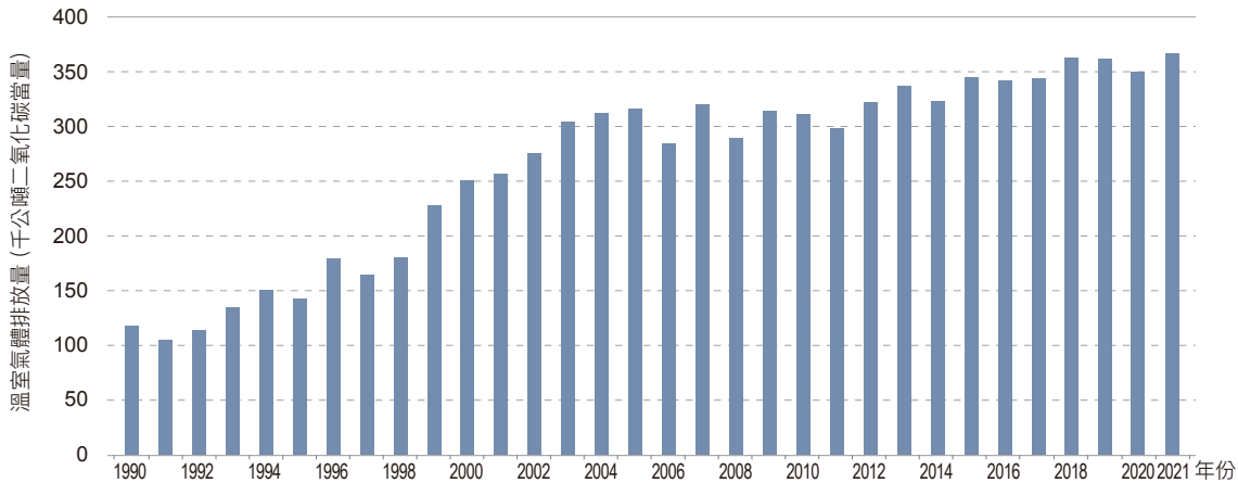
圖 4.3.9 1990 年至 2021 年氯乙烯生產製程排放量趨勢
