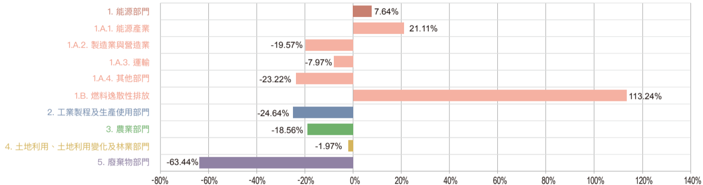
圖 ES3.3 2005 年至 2021 年各部門溫室氣體排放量和移除量變化
