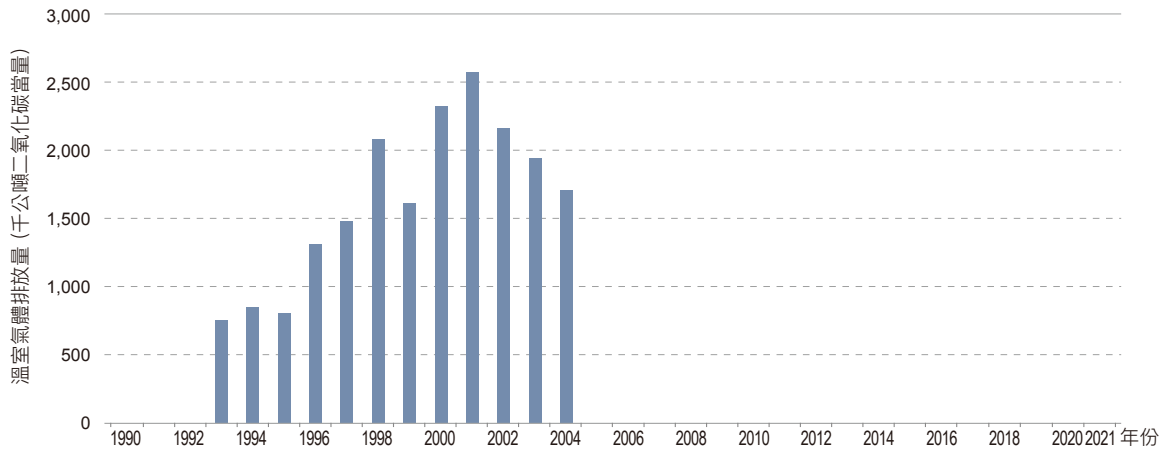
圖 4.3.13 1990 年至 2021 年 HCFC-22 副產品 (HFC-23) 排放量趨勢
