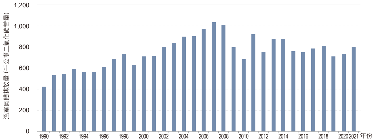
圖 4.4.3 1990 年至 2021 年電弧爐鋼胚生產製程排放量趨勢
