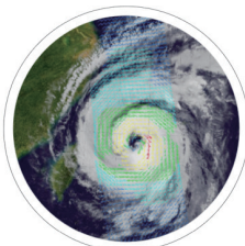
近海面風向風速
