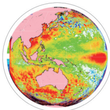
海表面溫度距平
