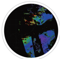
氣膠光學厚度
