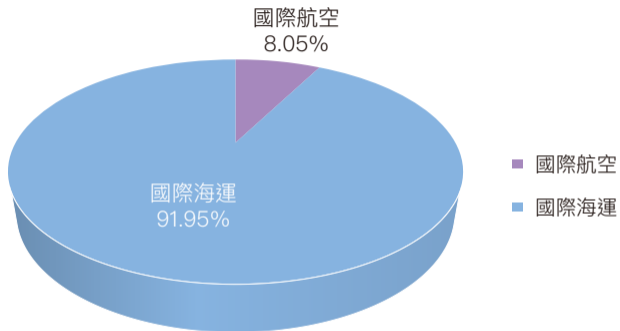
圖 3.2.35 2021 年國際運輸燃料燃燒甲烷排放占比
