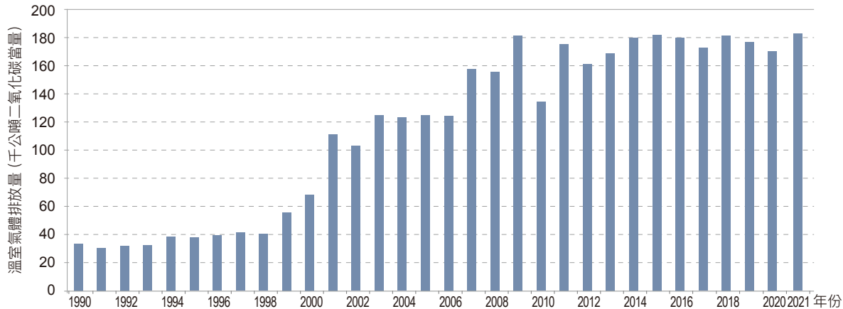
圖 4.3.8 1990 年至 2021 年乙烯生產製程排放量趨勢
