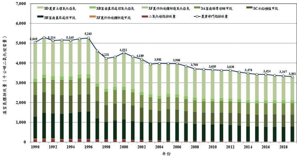
圖 2.4.3-1、臺灣 1990 至 2019 年農業部門溫室氣體排放量趨勢
