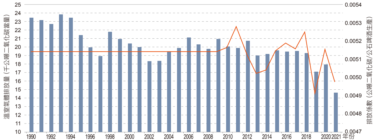
圖 4.9.1 1990 年至 2021 年啤酒製程排放量及歷年排放係數
