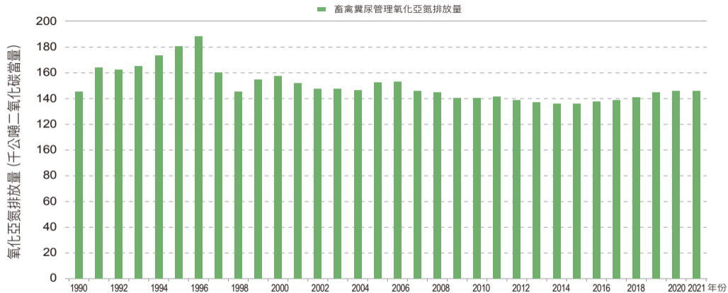
圖 5.3.2 1990 年至 2021 年畜禽糞尿管理之氧化亞氮排放量趨勢
