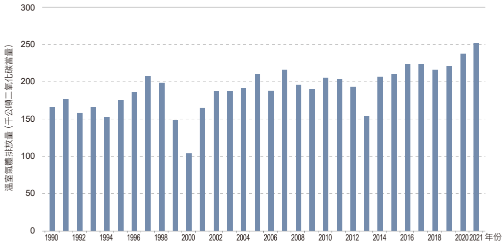
圖 4.3.2 1990 年至 2021 年硝酸生產製程排放量趨勢
