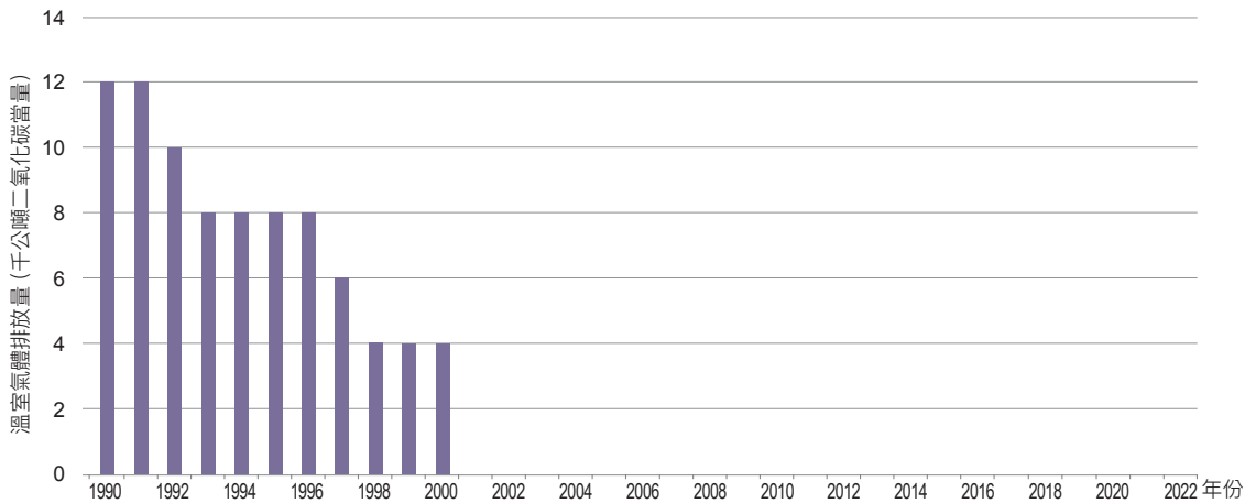
圖 4.3.6 1990 年至 2022 年純鹼生產製程排放量趨勢
