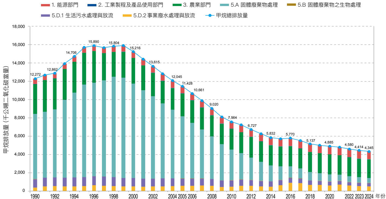
圖 2.2.2 1990 年至 2024 年甲烷排放量趨勢
