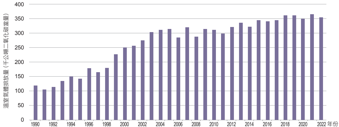
圖 4.3.9 1990 年至 2022 年氯乙烯生產製程排放量趨勢
