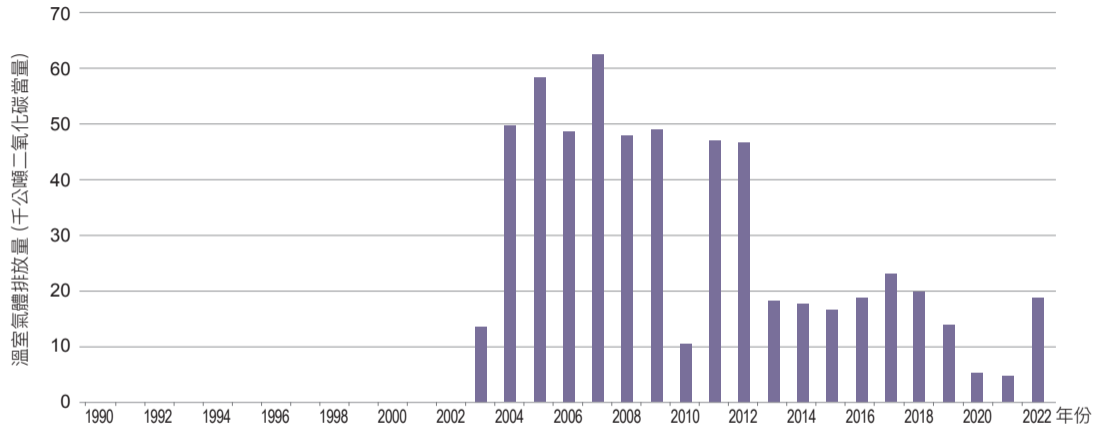
圖 4.4.8 1990 年至 2022 年鋅生產製程排放量趨勢
