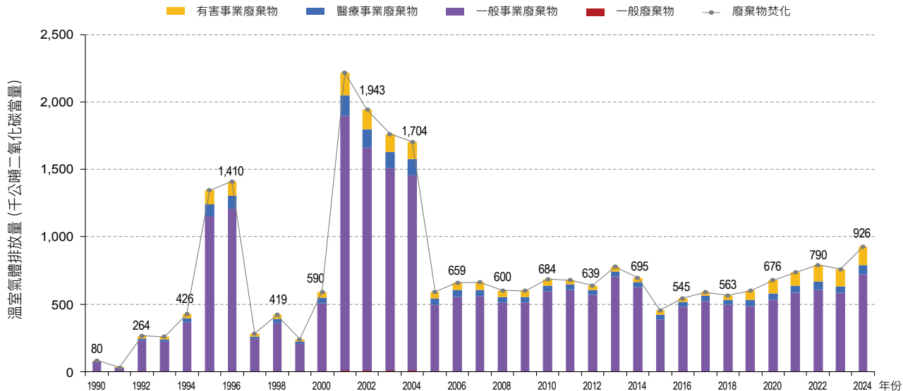
圖 7.4.1 1990 年至 2024 年廢棄物焚化溫室氣體排放量趨勢
