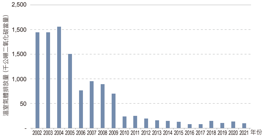
圖 4.8.1 2002 年至 2021 年電力設備中之六氟化硫排放趨勢
