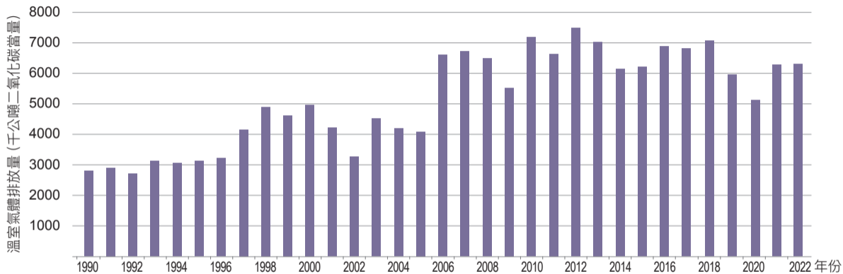
圖 4.4.2 1990 年至 2022 年高轉爐鋼胚生產製程排放量趨勢
