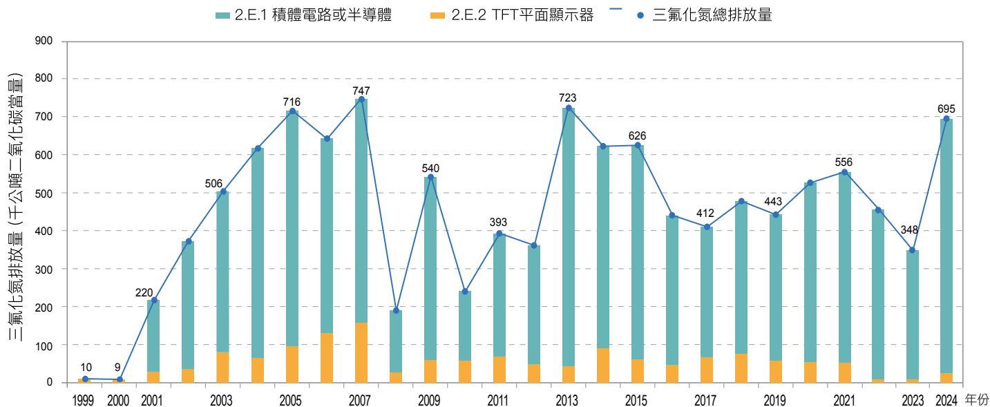
圖 2.2.7 1999 年至 2024 年三氟化氮排放量趨勢
