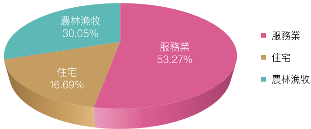
圖 3.2.31 2023 年服務業、住宅、農林漁牧燃料燃燒氧化亞氮排放占比
