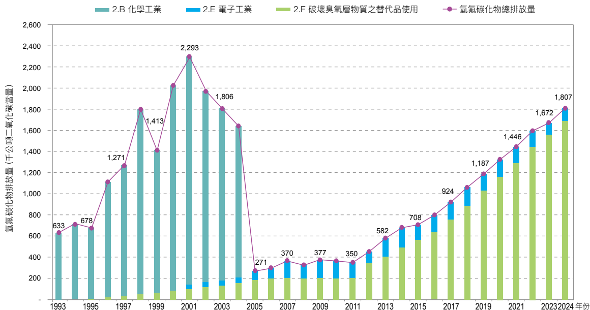
圖 2.2.4 1993 年至 2024 年氫氟碳化物排放量趨勢
