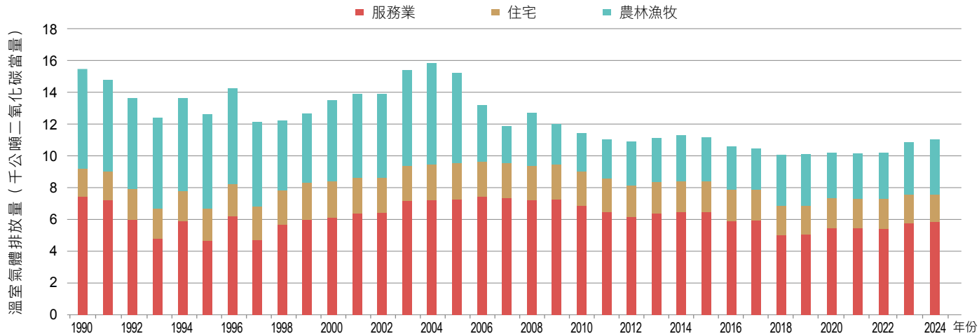
圖 3.2.39 1990 年至 2024 年服務業、住宅、農林漁牧燃料燃燒氧化亞氮排放量趨勢
