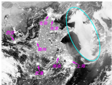
圖 6.2- 3 2023 年 3 月 10 日 ( 農曆 2 月 19 日 ) 凌晨 2 時 19 分中央氣象署接收繞極衛星 (SNPP) 觀測直接廣播，由左至右顯示日夜光頻道影像、日夜光與紅外線組合成的多頻道合成圖以及紅外線色調強化雲圖。左及中圖藍色圈圍可明顯見到黃海到東海的大範圍海霧；而陸地上的晴空區可見明顯的城市燈光。
