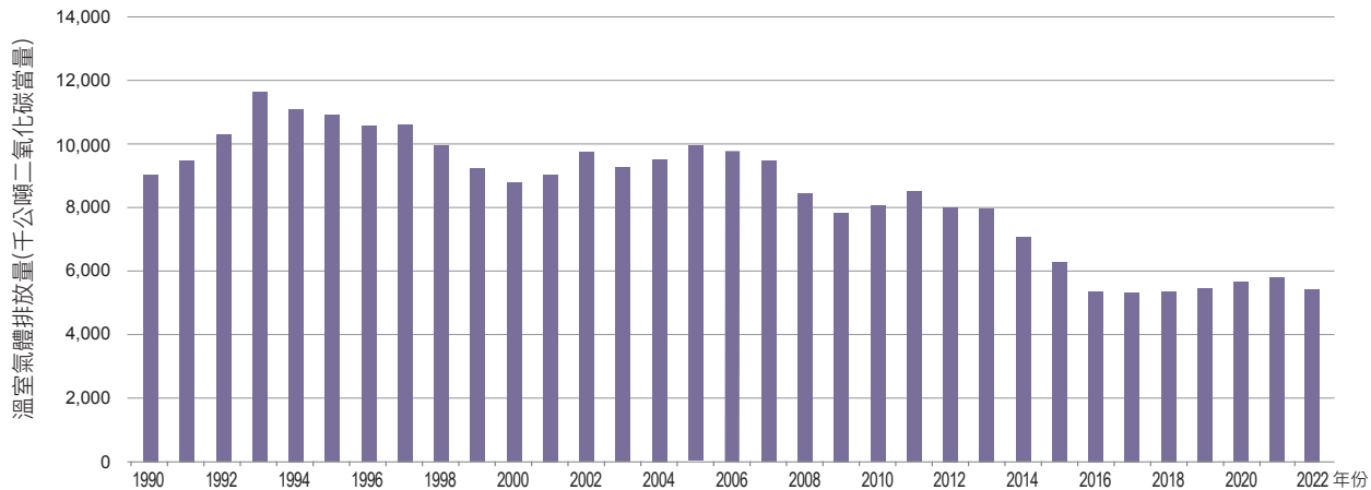
圖 4.2.2 1990 年至 2022 年水泥生產製程排放量趨勢
