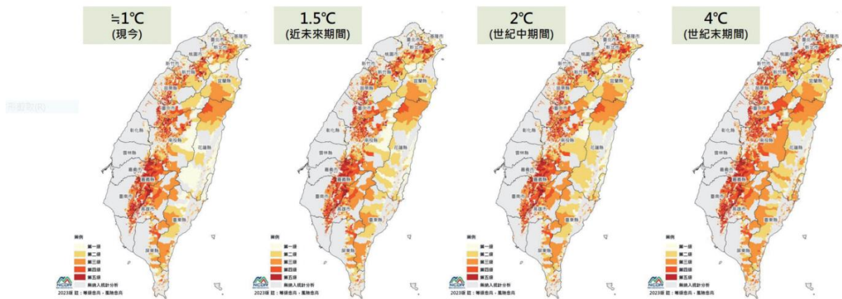
圖 14、全球暖化程度不同情境下最小人口統計區之坡地災害風險
