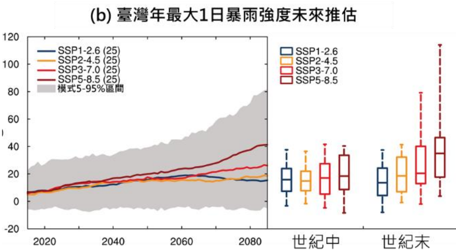
圖 25、臺灣未來年最大 1 日暴雨空間分布與強度推估
