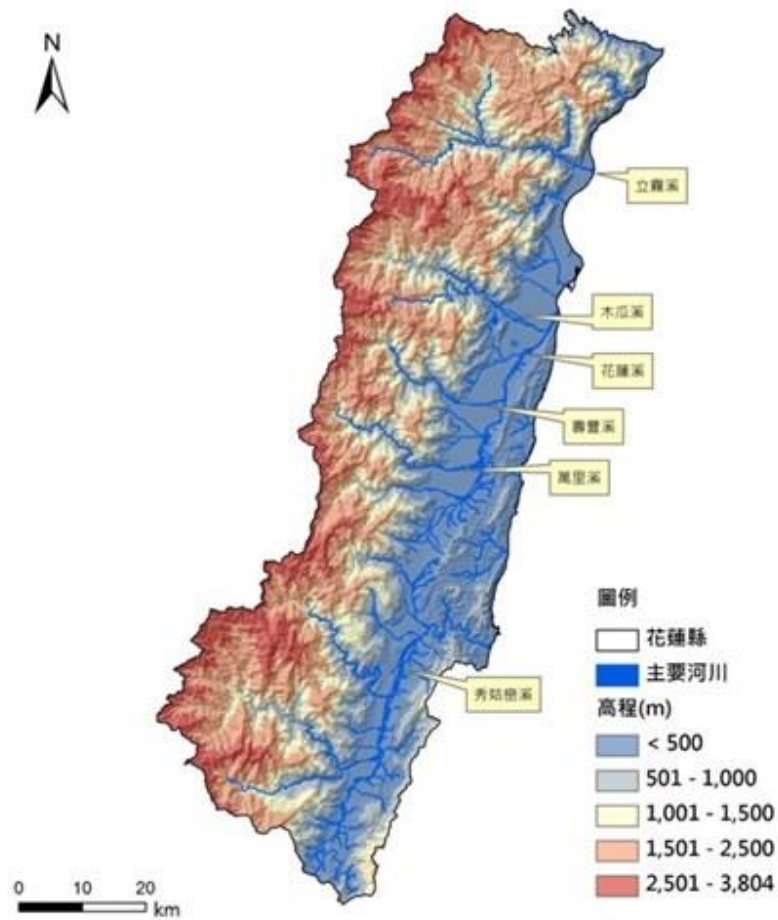
圖 2、花蓮縣地形、高程及水系分布圖
