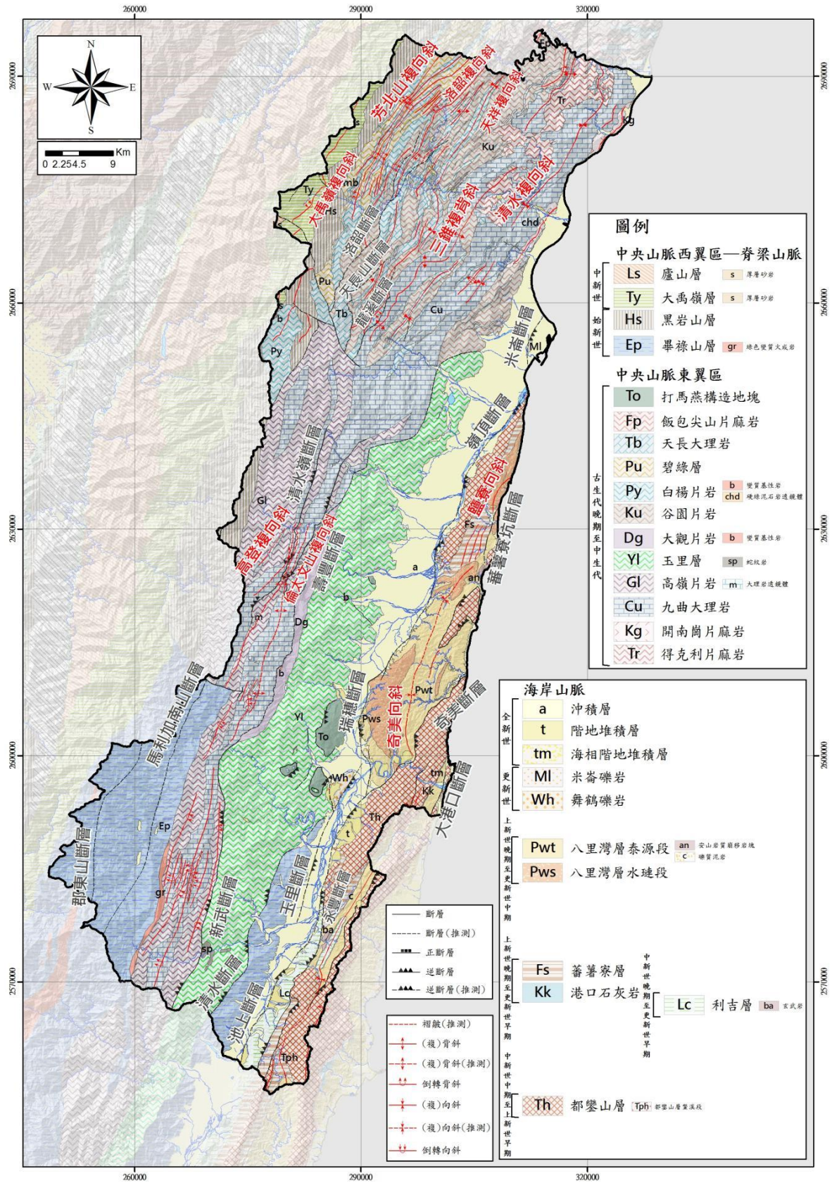
圖 3、花蓮縣地質圖
