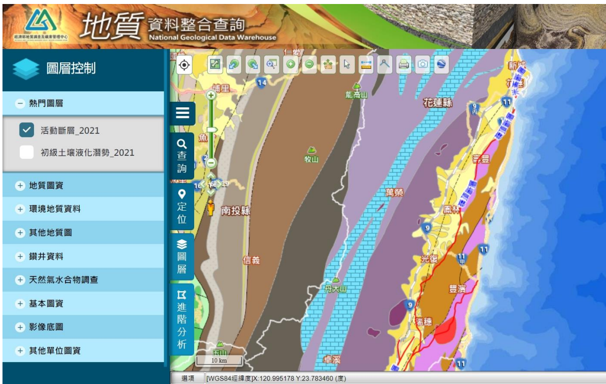
圖 12、花蓮縣主要斷層分布圖
