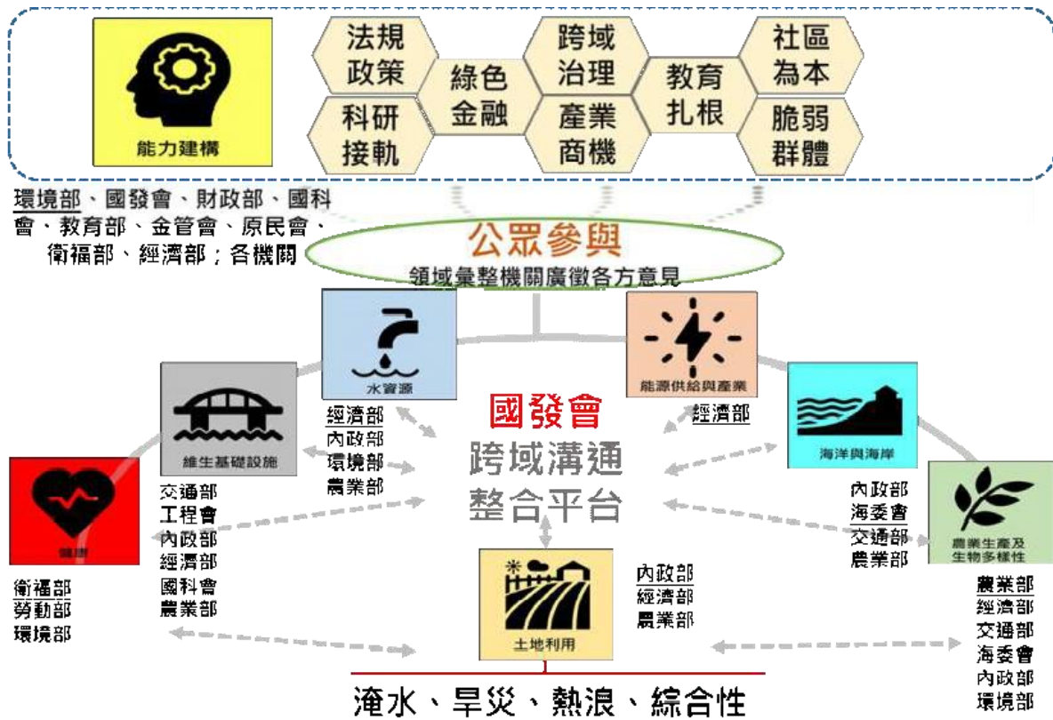
圖 17、國家氣候變遷調適領域架構
