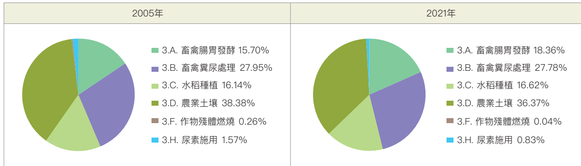
圖 ES3.6 2005 年和 2021 年農業部門溫室氣體排放量占比
