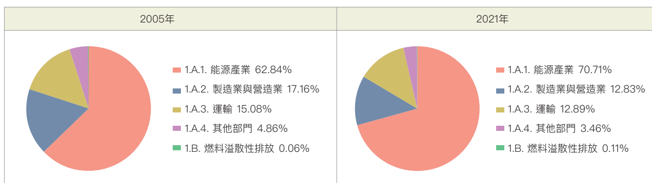
圖 ES3.4 2005 年和 2021 年能源部門溫室氣體排放量占比
