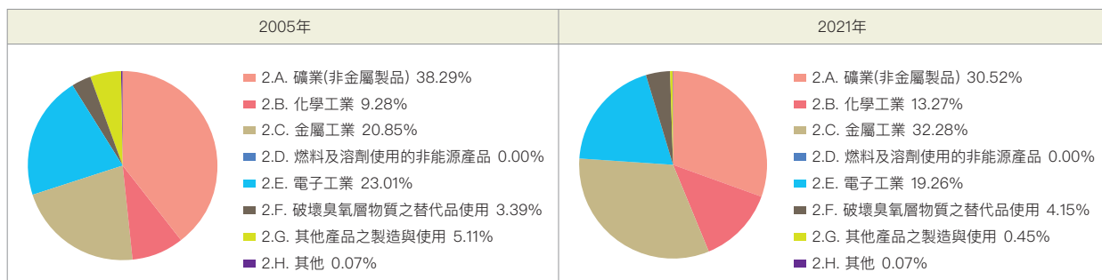
圖 ES3.5 2005 年和 2021 年工業製程及產品使用部門溫室氣體排放量占比
