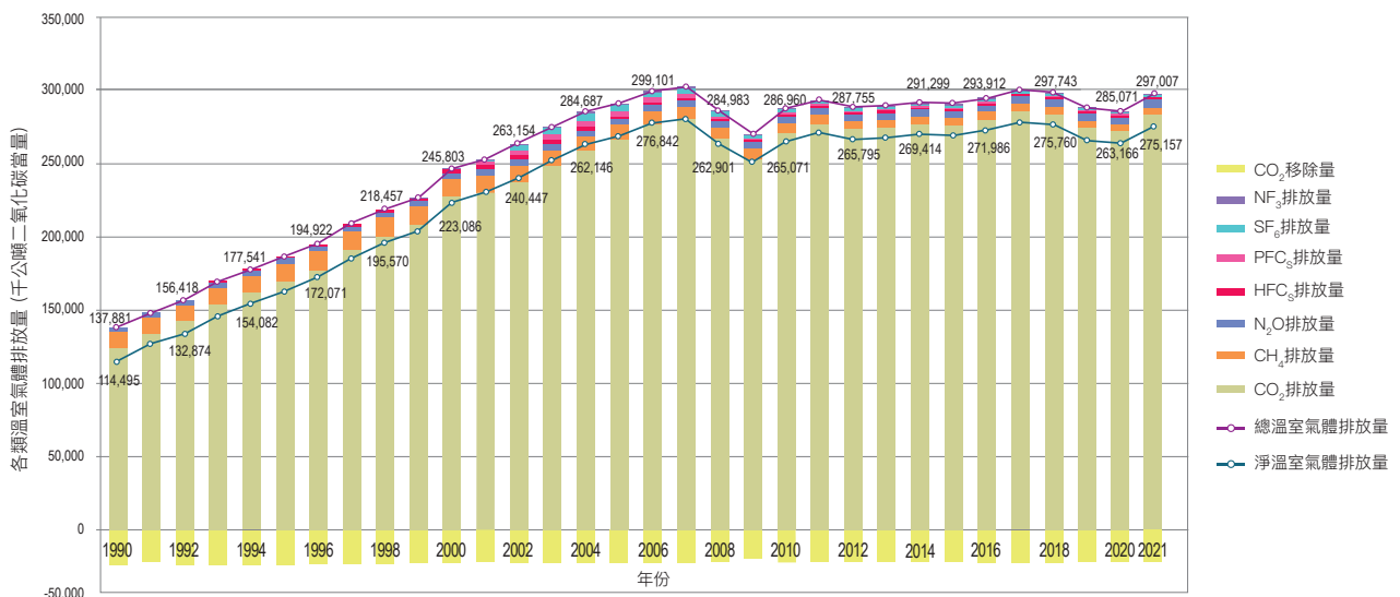
圖 ES2.3 1990 年至 2021 年各類溫室氣體排放量和移除量趨勢
