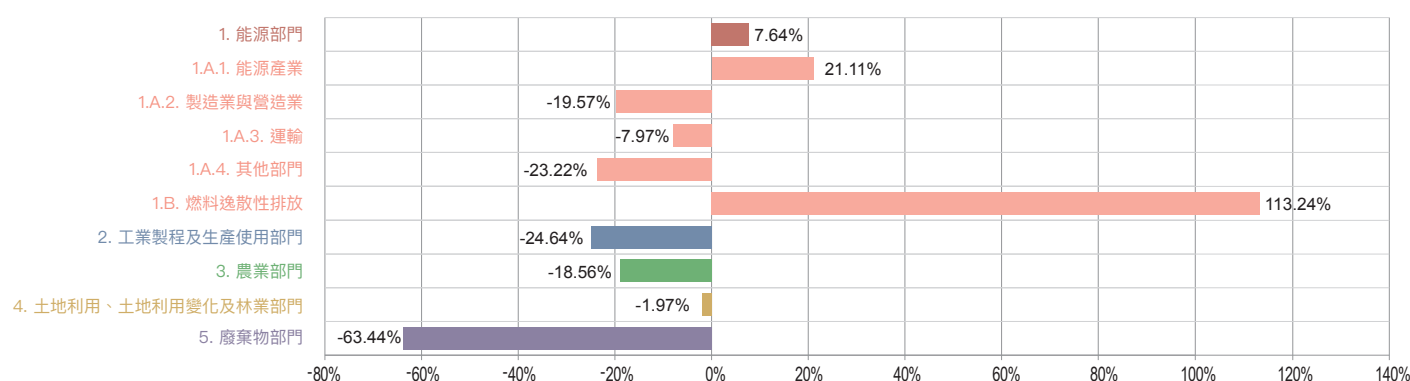
圖 ES3.3 2005 年至 2021 年各部門溫室氣體排放量和移除量變化
