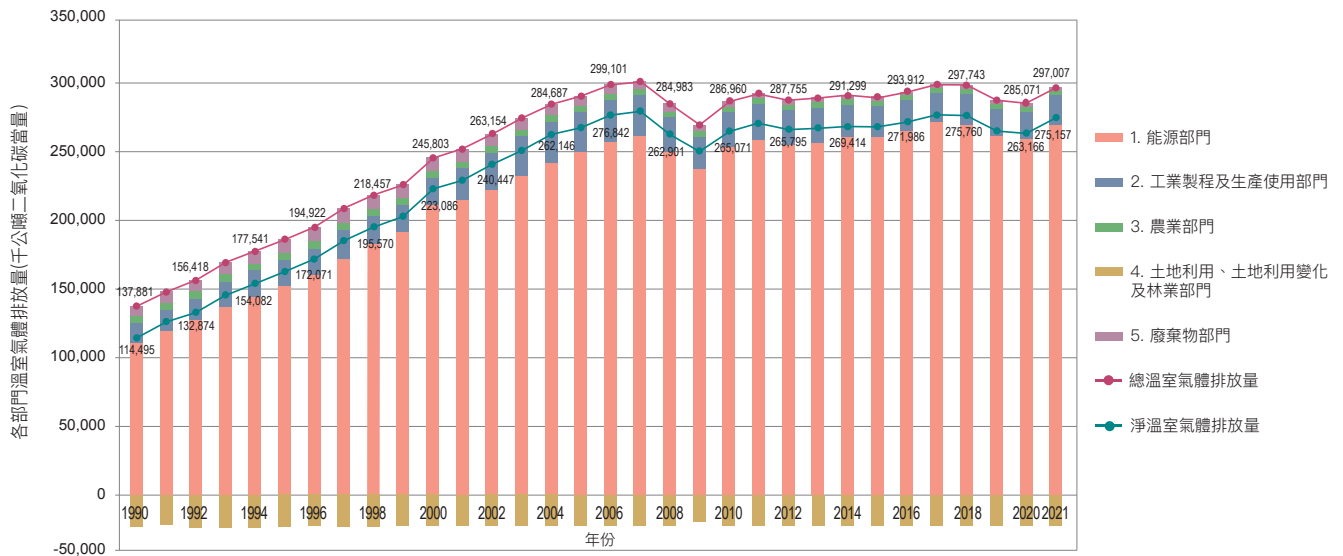
圖 ES3.2 1990 年至 2021 年各部門溫室氣體排放量趨勢
