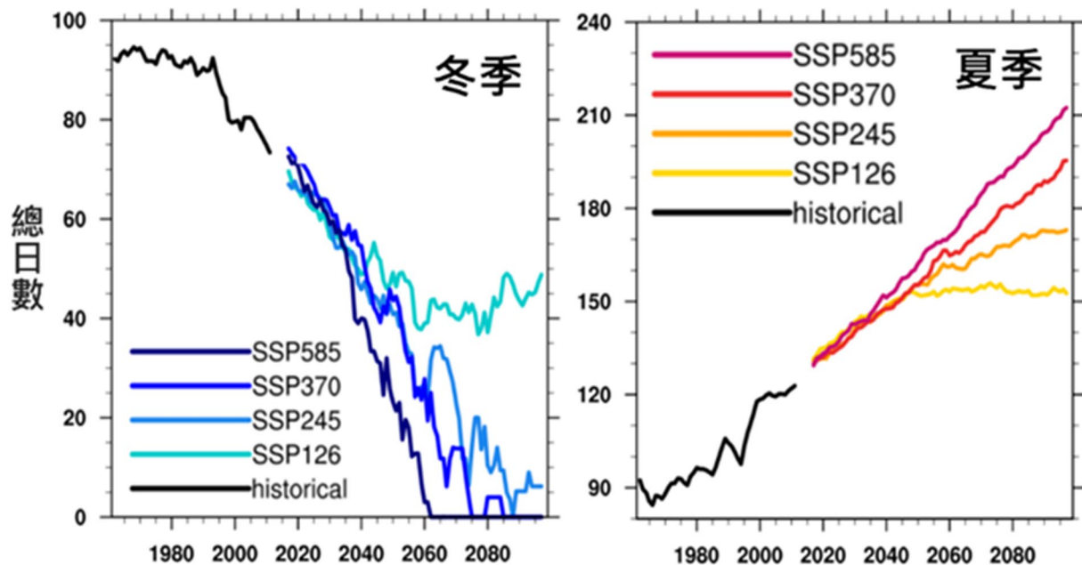
圖 5.1.1- 4 臺灣 ( 左 ) 冬季與 ( 右 ) 夏季長度的歷史與未來變化模擬 ( CMIP6 氣候模式 )
