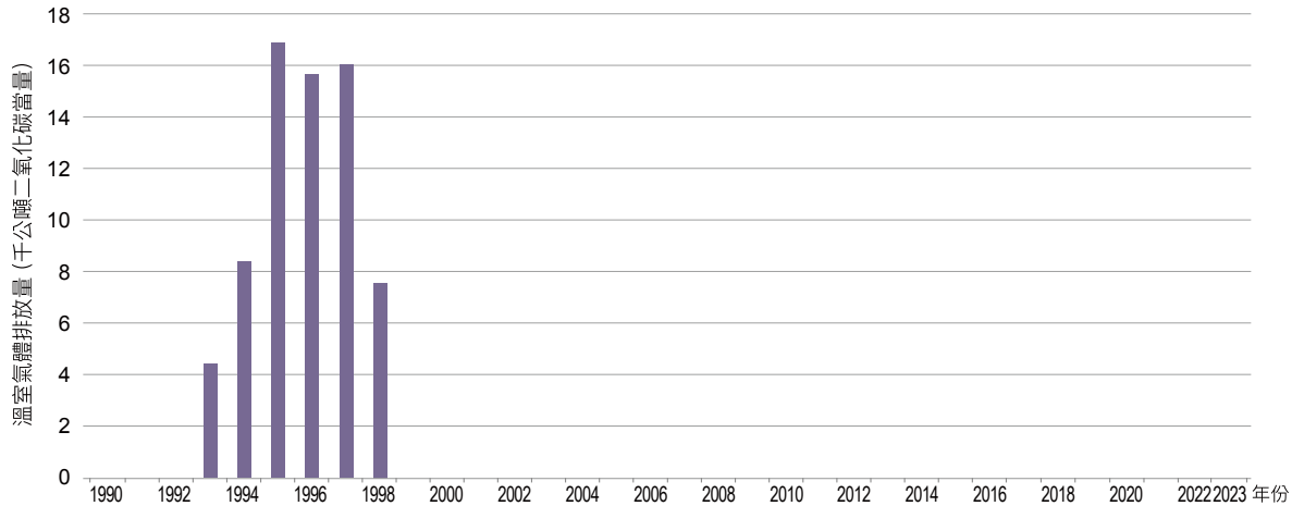
圖 4.3.7 1990 年至 2023 年甲醇生產製程排放量趨勢
