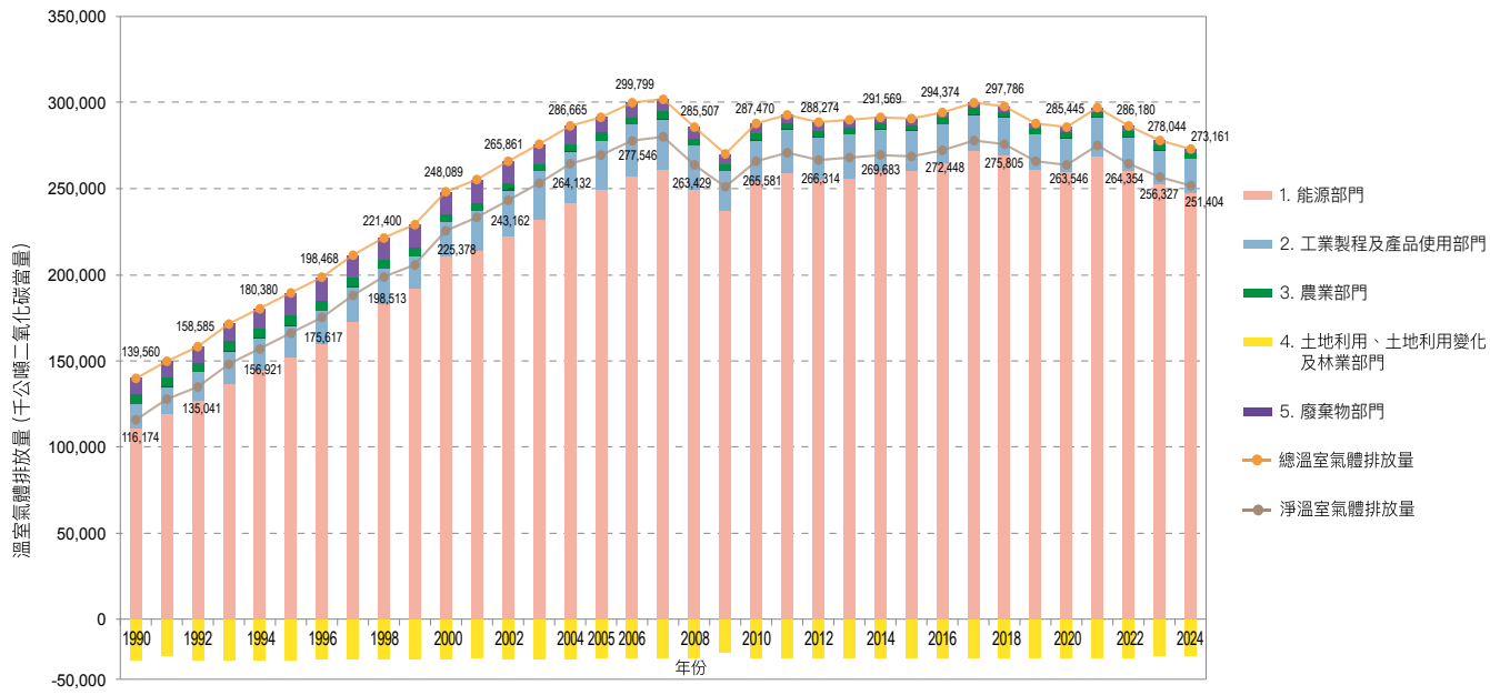
圖 ES3.2 1990 年至 2024 年各部門溫室氣體排放量趨勢
