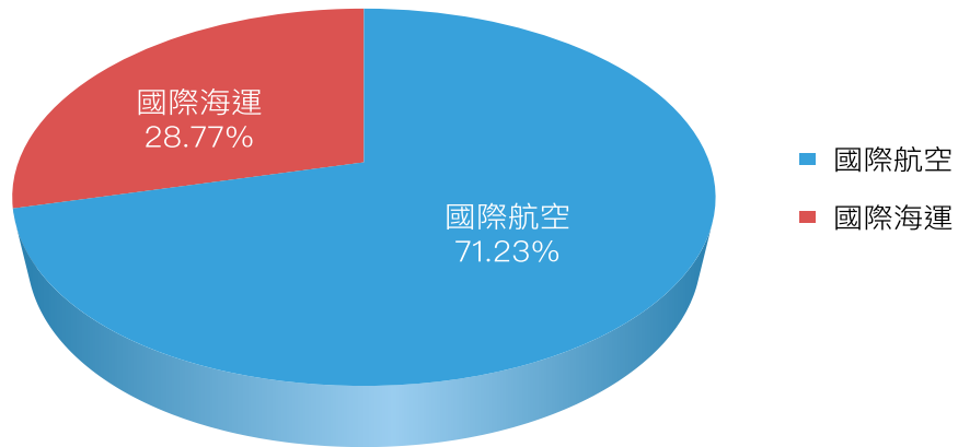
圖 3.2.13 2024 年國際運輸料燃燒各排放源氧化亞氮排放占比
