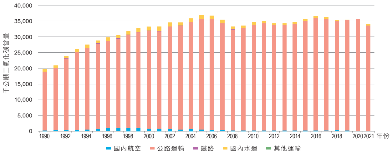
圖 3.2.20 1990 年至 2021 年運輸燃料燃燒二氧化碳排放量趨勢
