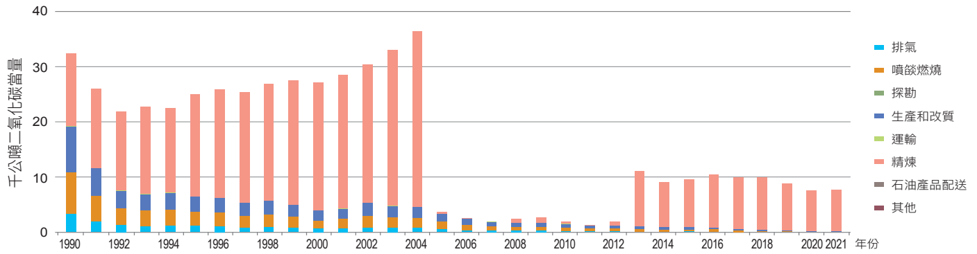
圖 3.3.5 1990 年至 2021 年石油逸散溫室氣體排放量趨勢
