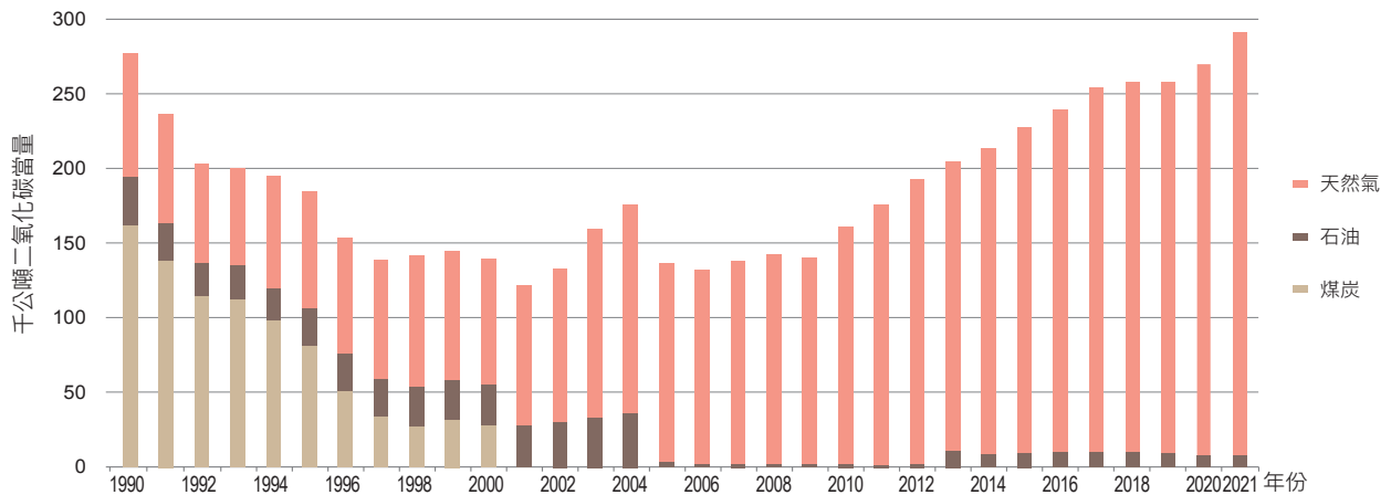
圖 3.3.1 1990 年至 2021 年能源部門燃料逸散溫室氣體排放量趨勢
