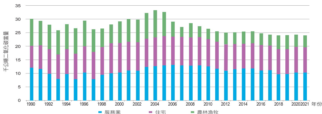
圖 3.2.28 1990 年至 2021 年服務業、住宅、農林漁牧燃料燃燒甲烷排放量趨勢
