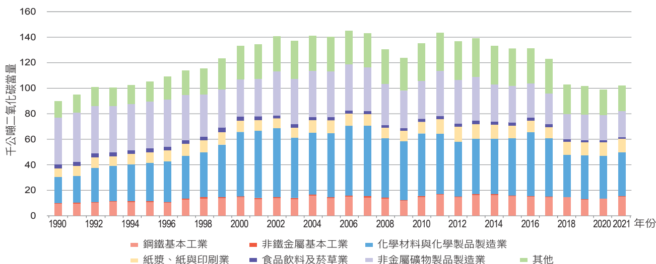
圖 3.2.16 1990 年至 2021 年製造業與營造業燃料燃燒甲烷排放量趨勢
