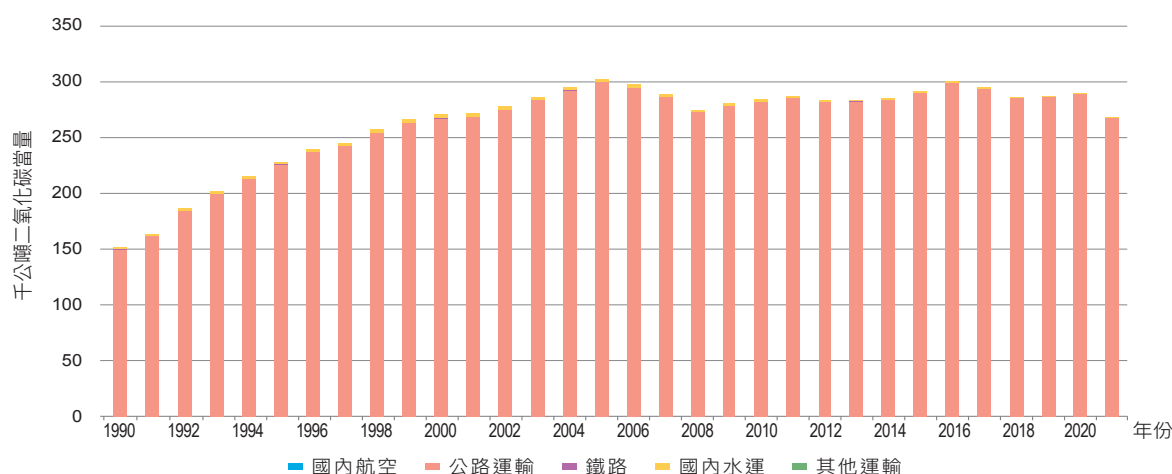
圖 3.2.22 1990 年至 2021 年運輸燃料燃燒甲烷排放量趨勢
