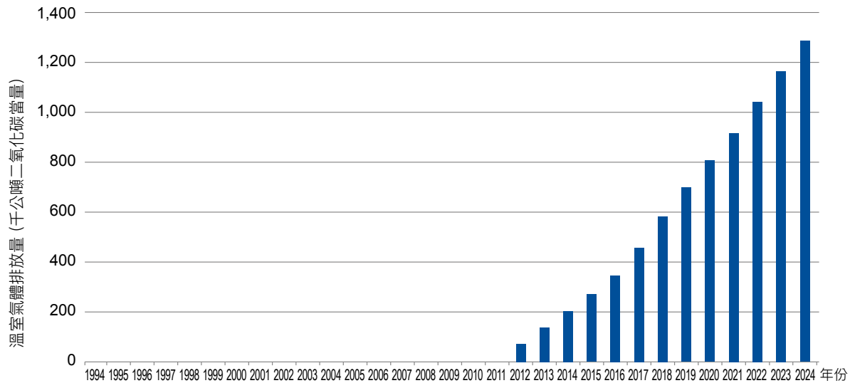
圖 4.7.4 1994 年至 2024 年固定式空調之 HFCs 排放量趨勢
