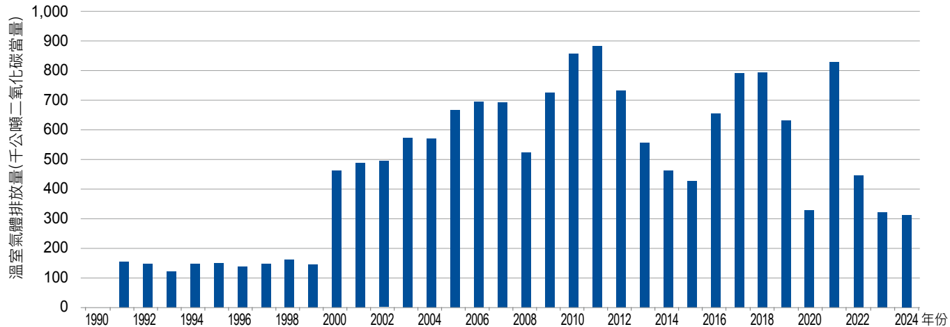
圖 4.3.3 1990 年至 2024 年己內醯胺生產製程排放量趨勢
