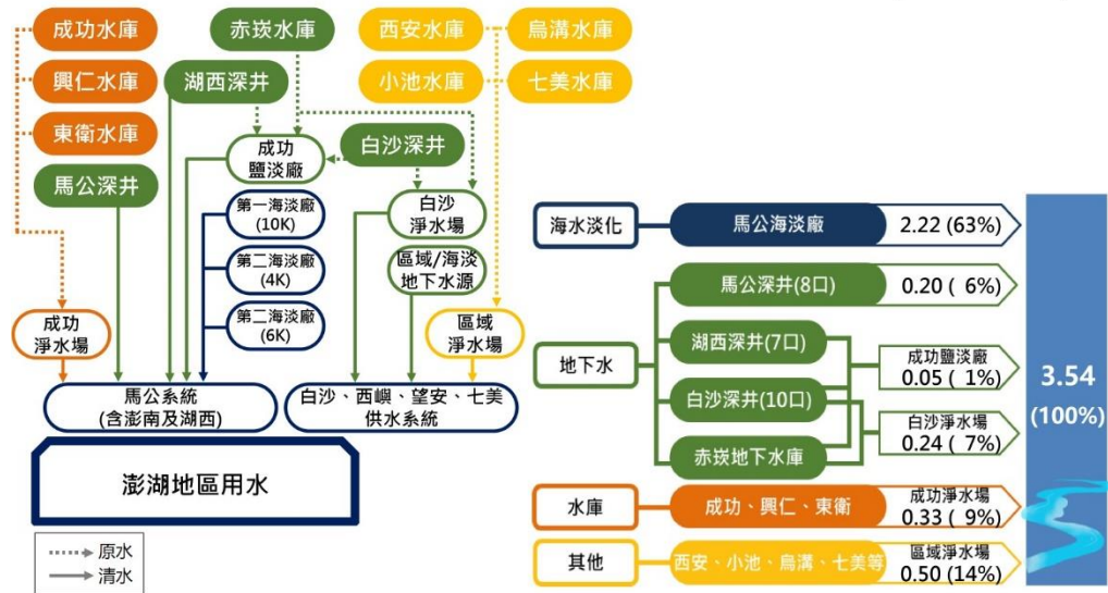
圖 2.8 澎湖地區自來水水源供需圖
