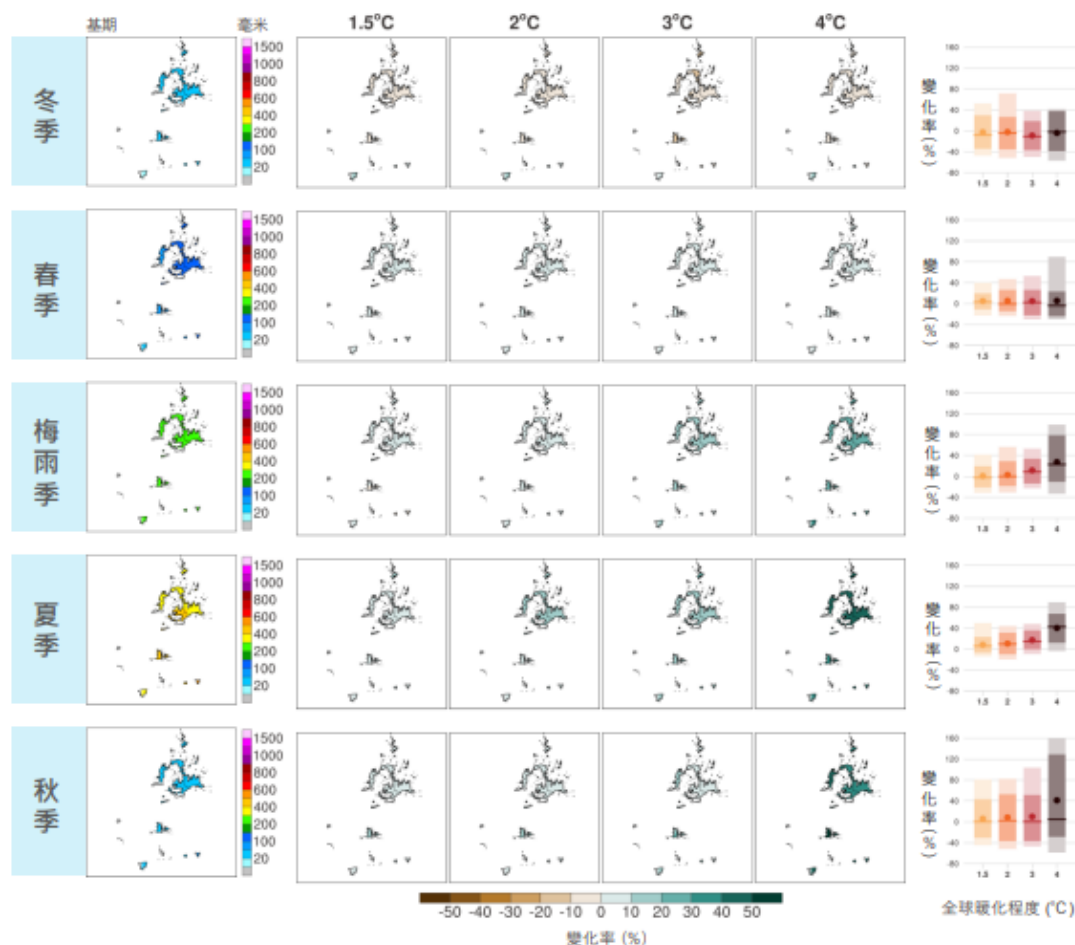
圖 2.31 澎湖縣未來季節降雨變化推估
