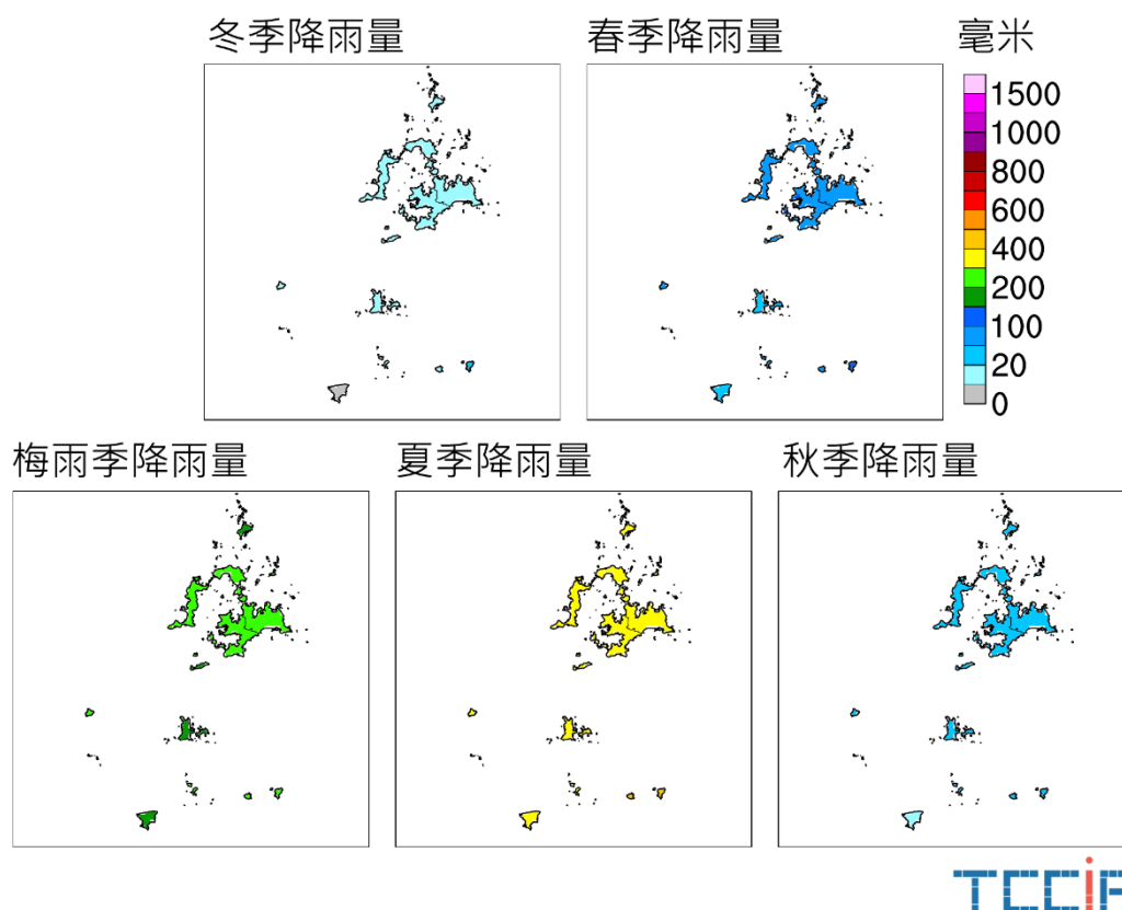
圖 2.15 澎湖縣季節降雨空間分布(1991-2020 年)
