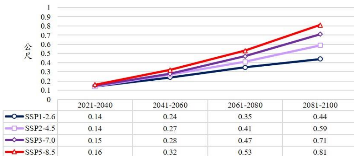
圖 2.32 澎湖縣未來海平面情景推估(SSP-RCPs)
