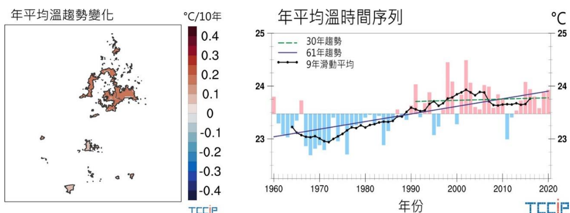
圖 2.16 澎湖年平均溫趨勢變化及時間序列(1960-2020 年)
