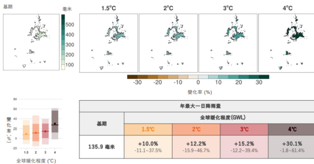
圖 2.29 澎湖縣未來年最大一日降雨量推估
