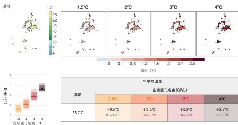
圖 2.26 澎湖縣未來年平均溫度趨勢推估
