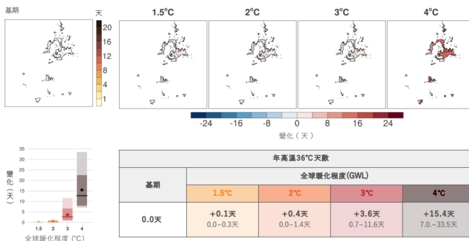
圖 2.27 澎湖縣未來年高溫 36°C 天數推估
