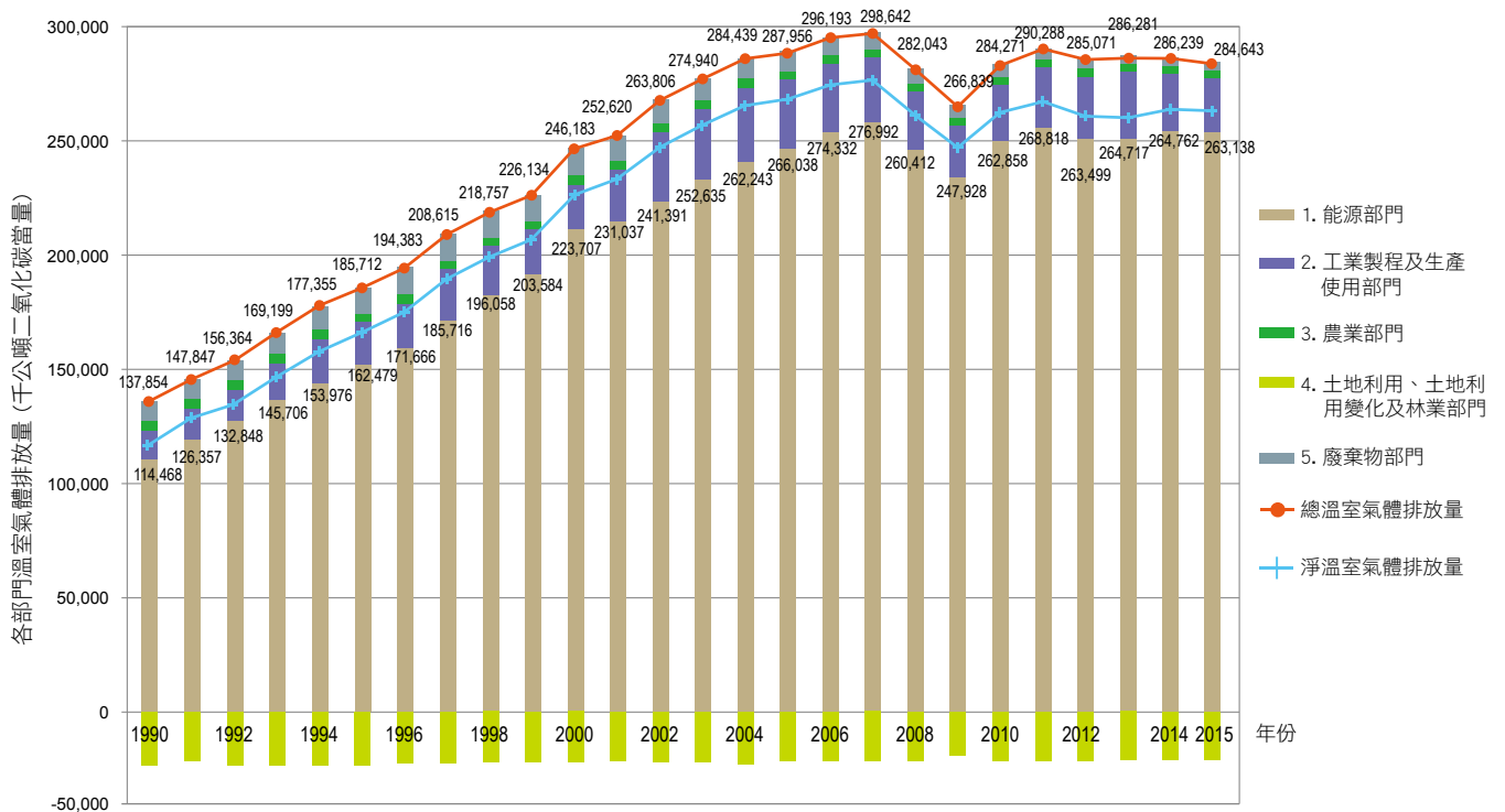
圖 ES3.1 臺灣 1990 至 2015 年各部門溫室氣體排放量趨勢
