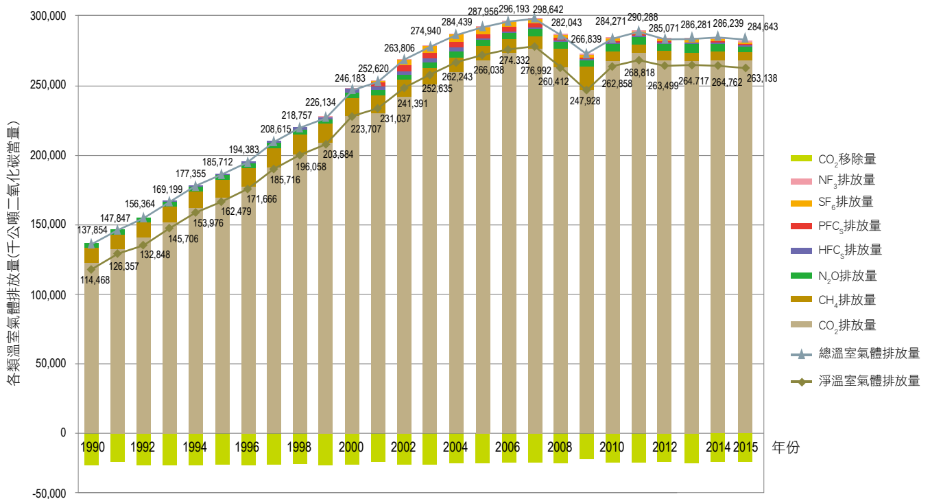
圖 ES2.1 臺灣 1990 至 2015 年總溫室氣體排放量和移除量趨勢
