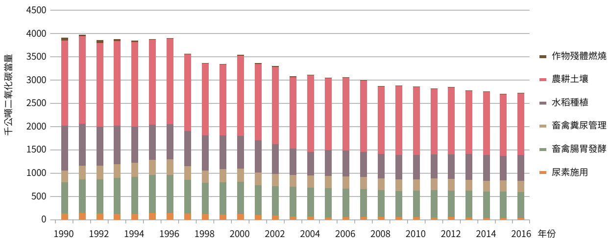
圖 5.1.1 臺灣 1990 至 2016 年農業部門排放量趨勢
