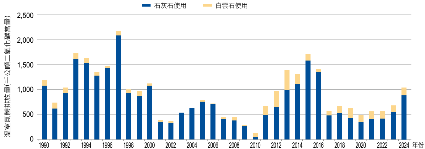
圖 4.2.8 1990 年至 2024 年石灰石與白雲石使用排放量趨勢
