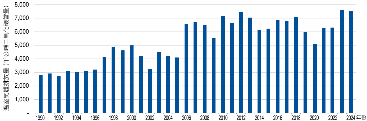
圖 4.4.2 1990 年至 2024 年高爐鋼胚生產製程排放量趨勢
