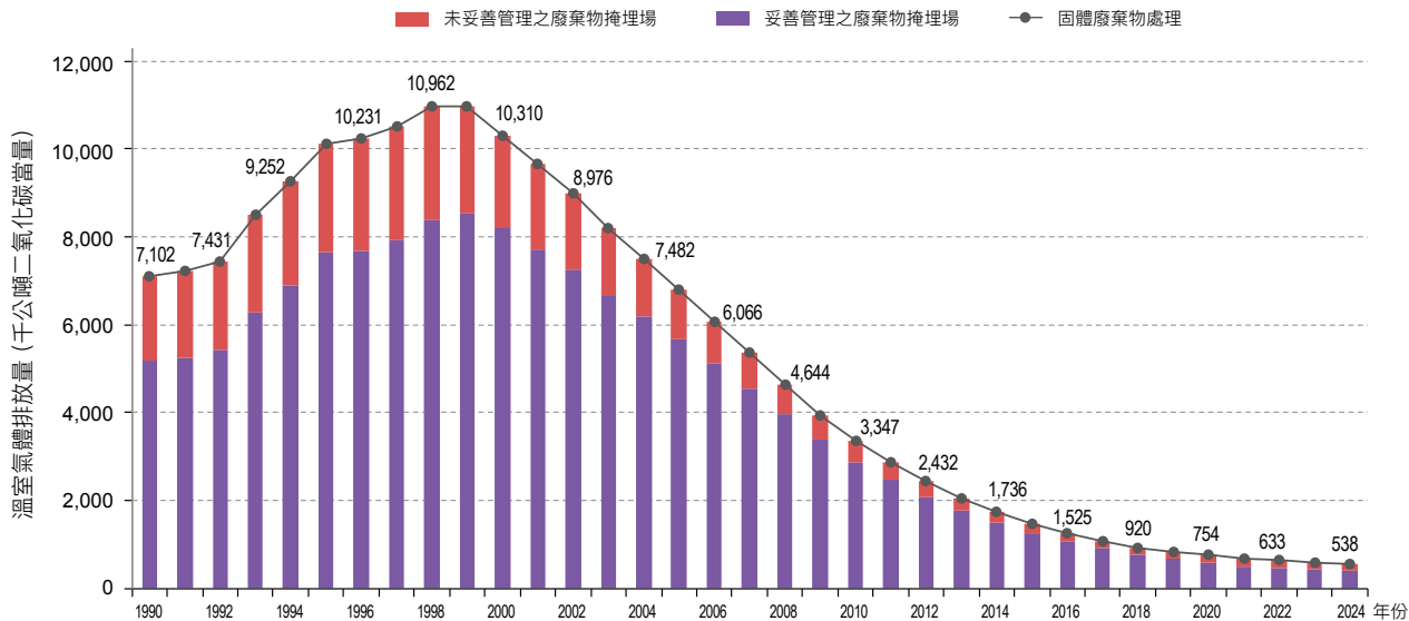
圖 7.2.1 1990 年至 2024 年固體廢棄物處理溫室氣體排放量趨勢
