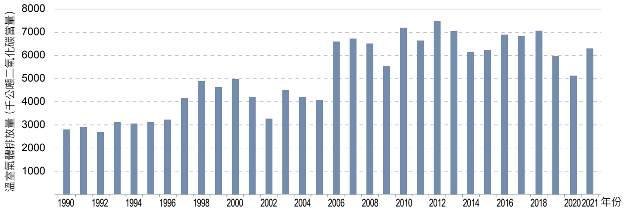
圖 4.4.2 1990 年至 2021 年高轉爐鋼胚生產製程排放量趨勢
