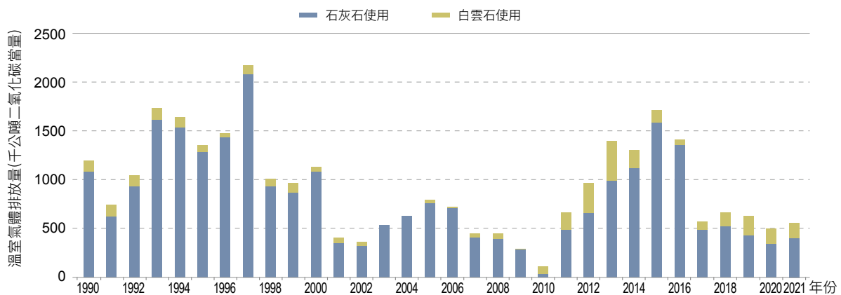
圖 4.2.7 1990 年至 2021 年石灰石與白雲石使用排放量趨勢
