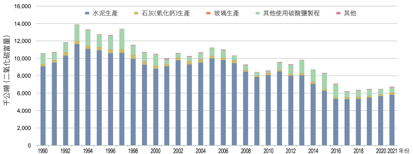
圖 4.2.1 1990 年至 2021 年礦業（非金屬工業）排放量趨勢
