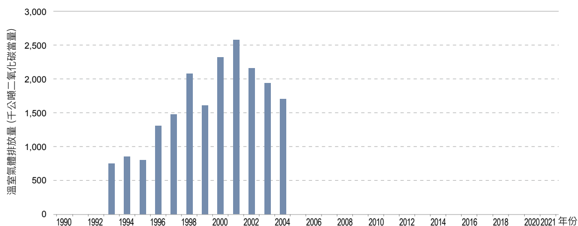
圖 4.3.13 1990 年至 2021 年 HCFC-22 副產品 (HFC-23) 排放量趨勢
