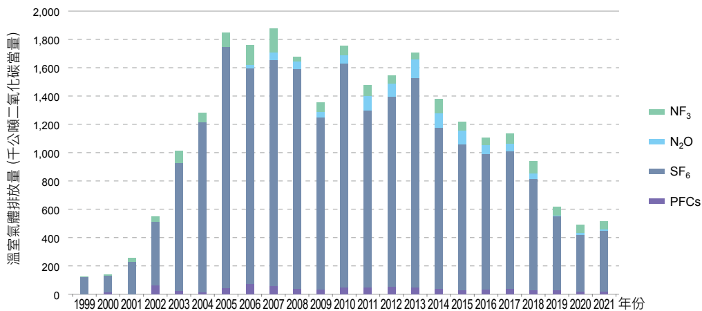
圖 4.6.4 1999 年至 2021 年 TFT 平面顯示器製程排放量趨勢
