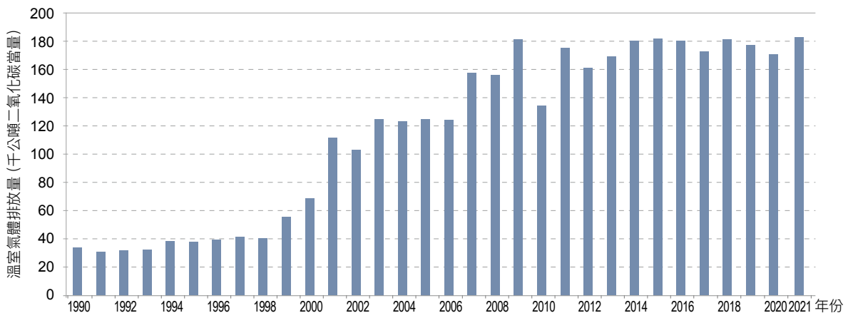
圖 4.3.8 1990 年至 2021 年乙烯生產製程排放量趨勢
