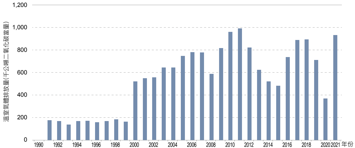
圖 4.3.3 1990 年至 2021 年己內醯胺生產製程排放量趨勢
