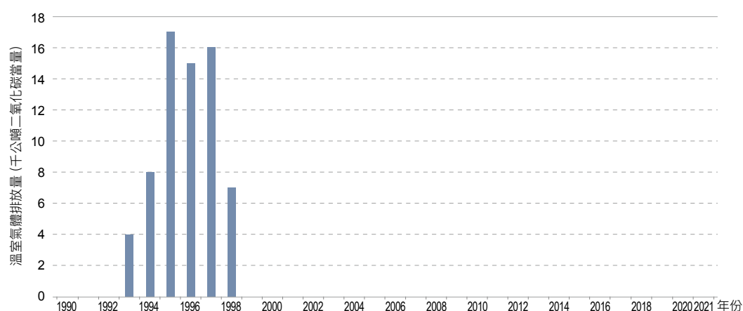
圖 4.3.7 1990 年至 2021 年甲醇生產製程排放量趨勢
