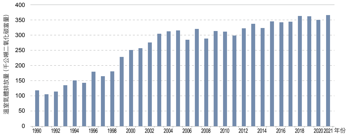
圖 4.3.9 1990 年至 2021 年氯乙烷生產製程排放量趨勢
