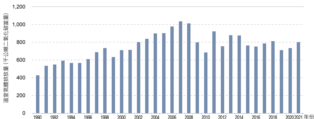
圖 4.4.3 1990 年至 2021 年電弧爐鋼胚生產製程排放量趨勢
