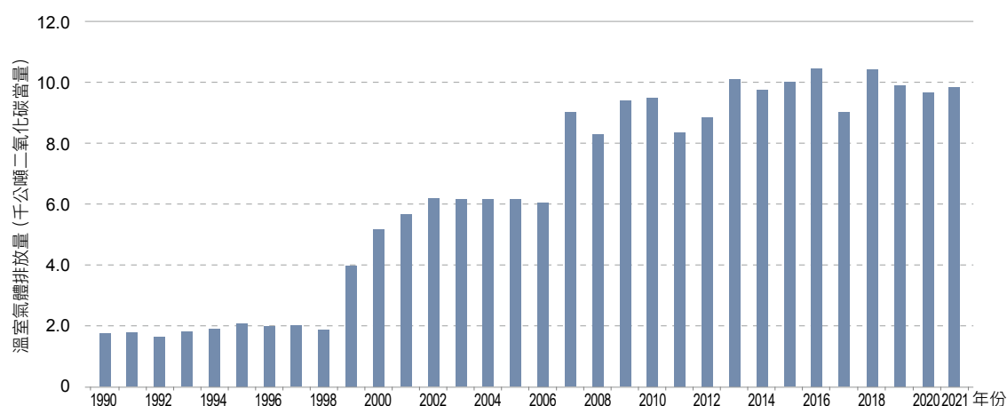
圖 4.3.14 1990 年至 2021 年苯乙烯生產製程排放量趨勢
