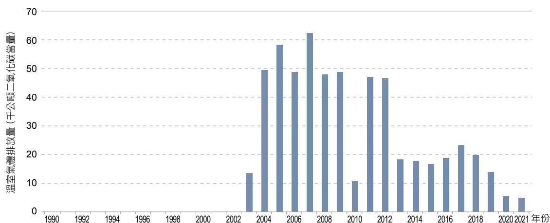
圖 4.4.8 1990 年至 2021 年鋅生產製程排放量趨勢
