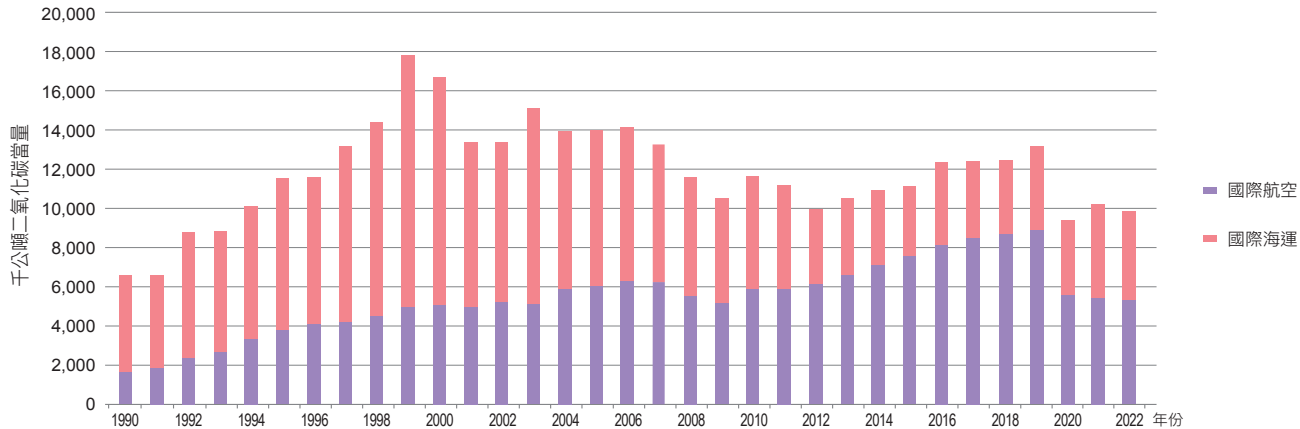
圖 3.2.32 1990 年至 2022 年國際運輸燃料燃燒二氧化碳排放量趨勢
