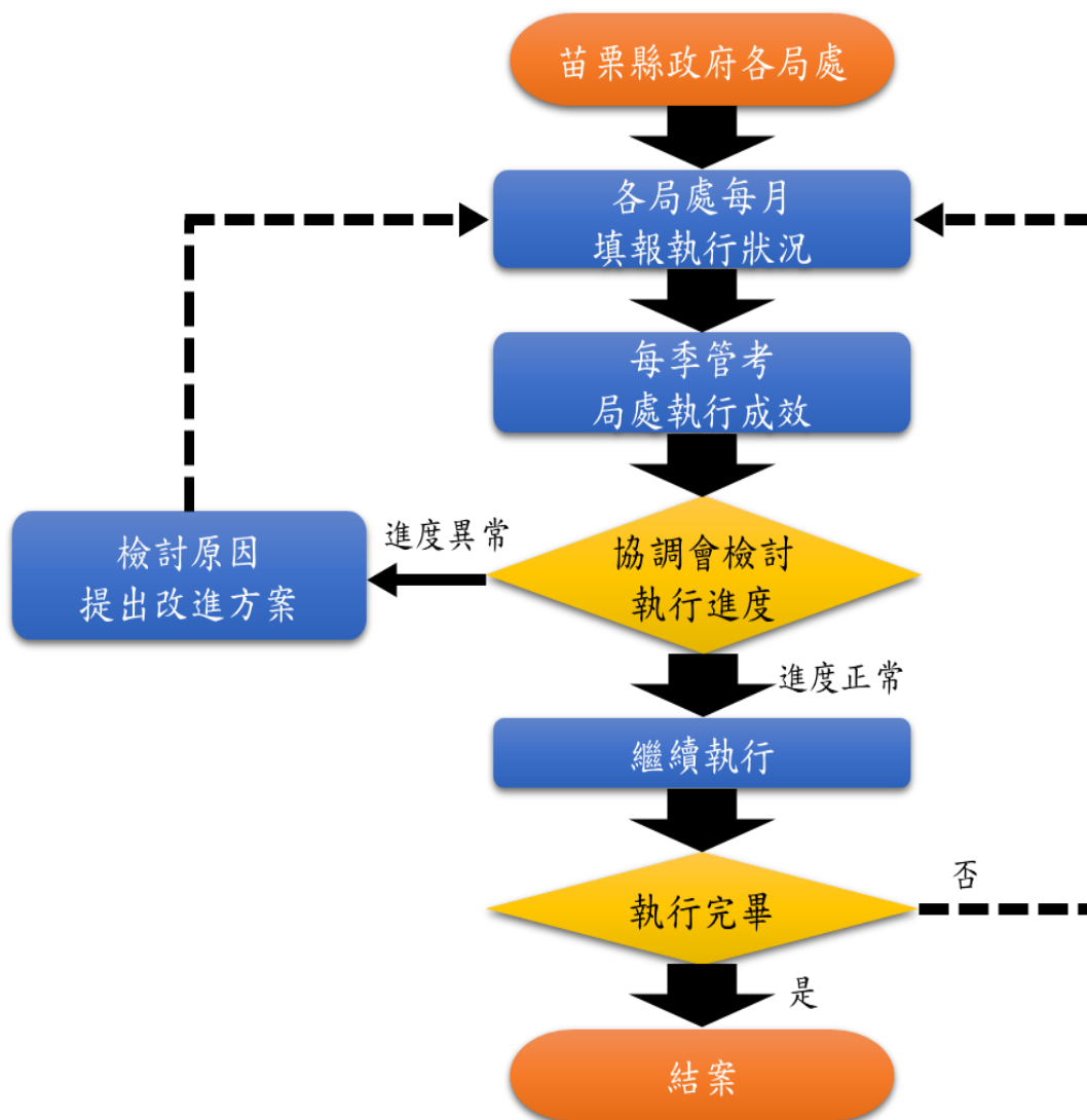
圖 6-1 管考流程圖
