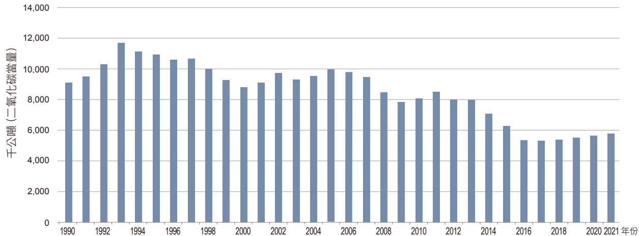
圖 4.2.2 1990 年至 2021 年水泥生產製程排放量趨勢
