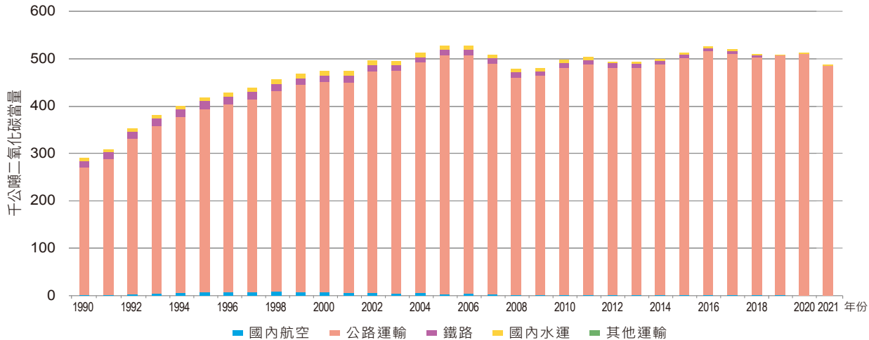
圖 3.2.24 1990 年至 2021 年運輸燃料燃燒氧化亞氮排放量趨勢
