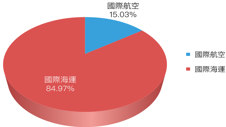
圖 3.2.11 2024 年國際運輸燃料燃燒各排放源甲烷排放占比
