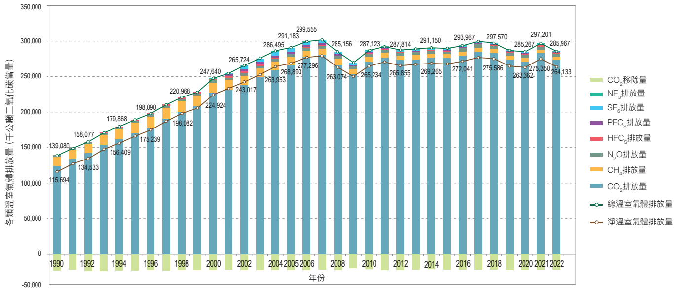
圖 2.1.1 1990 年至 2022 年總溫室氣體排放量和移除量趨勢
