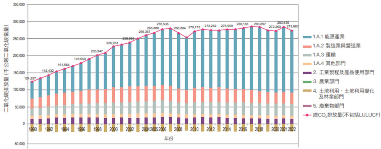
圖 2.3.1- 1 臺灣 1990 至 2022 年二氧化碳排放量趨勢
