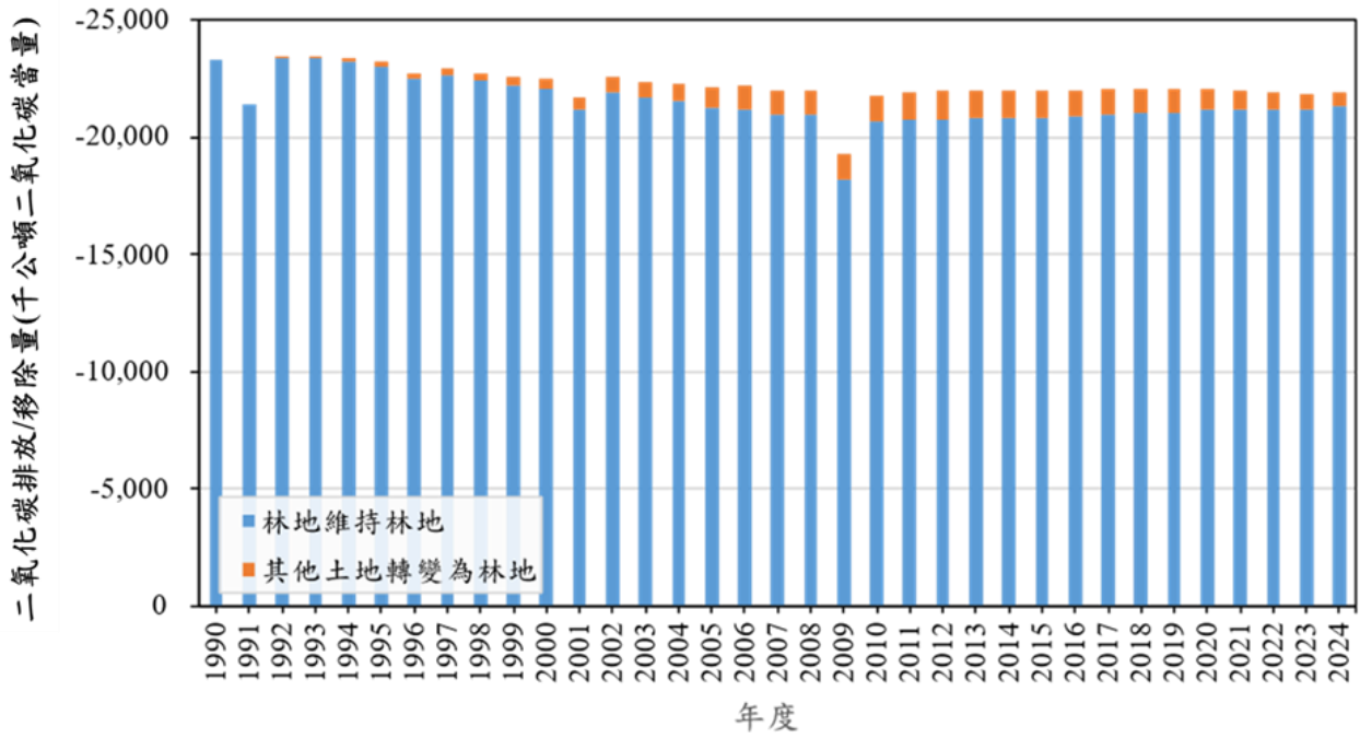
圖 6.2.1 1990 年至 2024 年林地碳移除量變化趨勢 (依類別)
