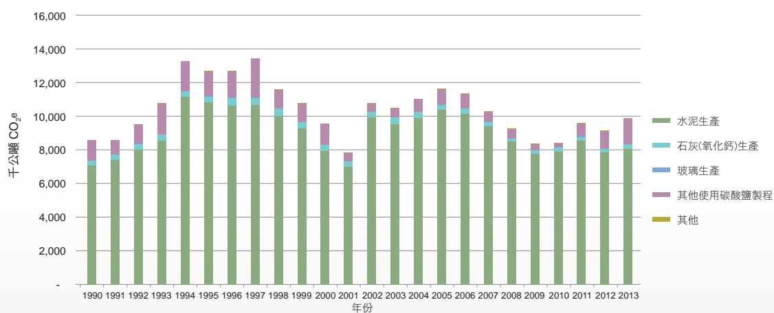
圖 4.2.1 臺灣 1990 至 2013 年礦業（非金屬製程）排放量趨勢
