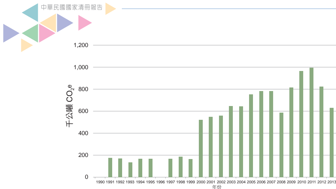
圖 4.3.4 臺灣 1990 至 2013 年己內醯胺生產排放量趨勢
