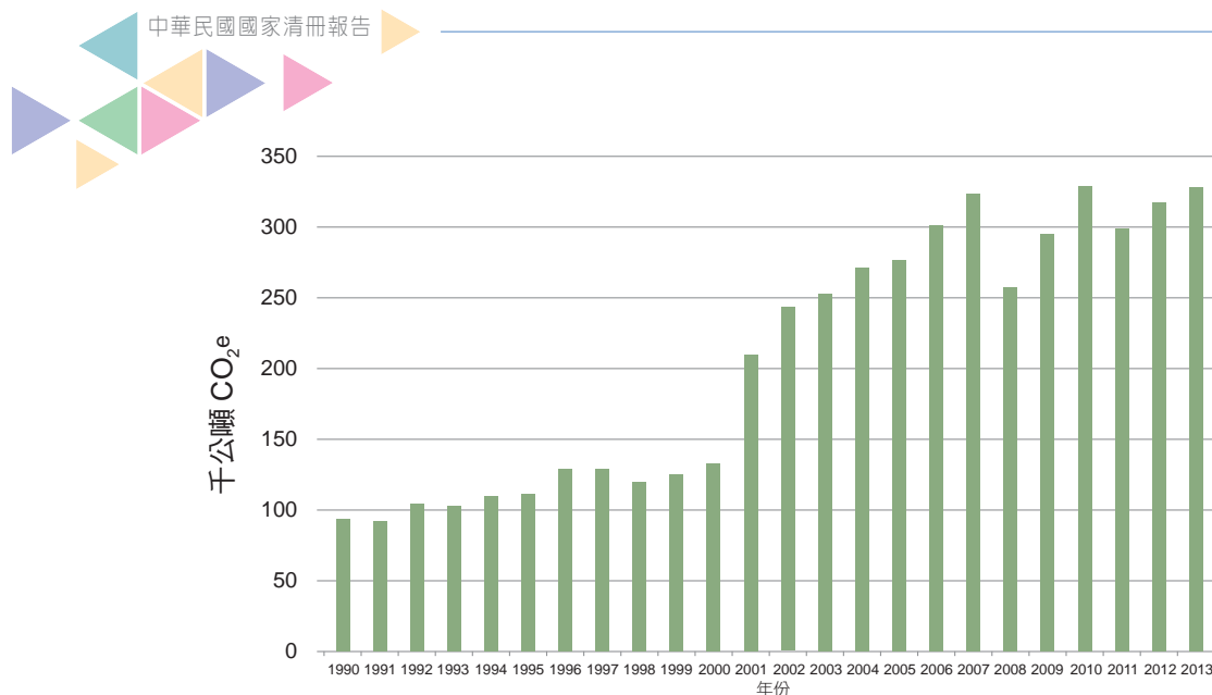
圖 4.3.12 臺灣 1990 至 2013 年丙烯腈生產排放量趨勢
