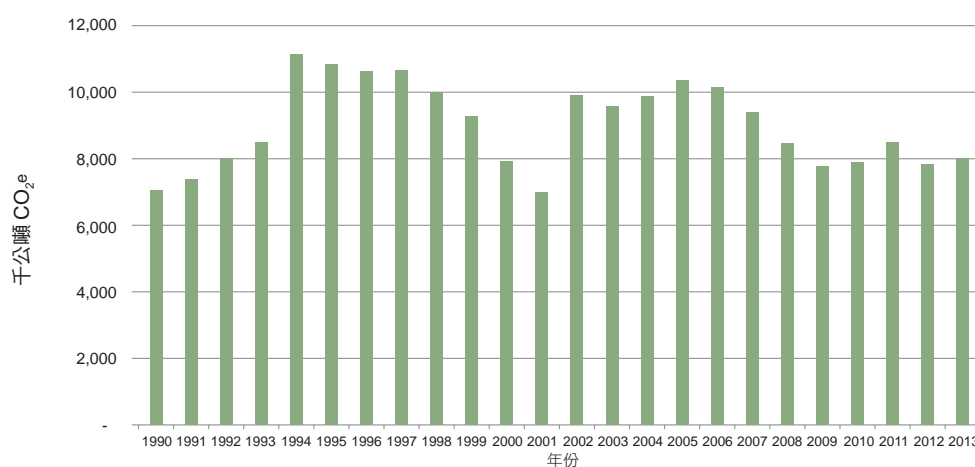
圖 4.2.2 臺灣 1990 至 2013 年水泥生產排放量趨勢
