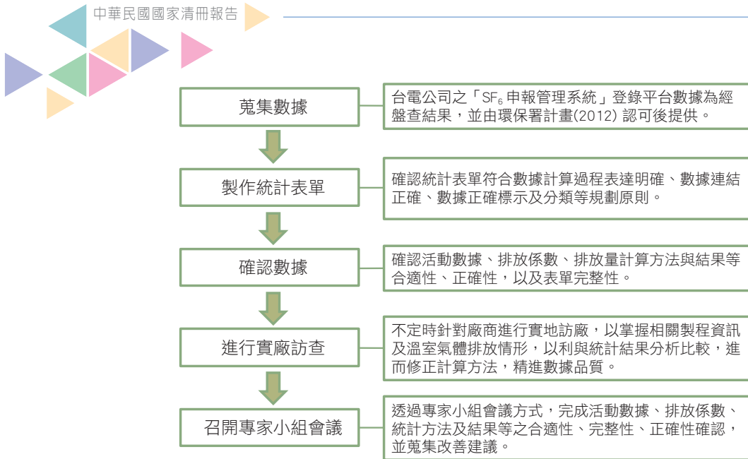
圖 4.8.2 高壓斷路器及其他開關絕緣氣體排放統計 QA/QC 流程
