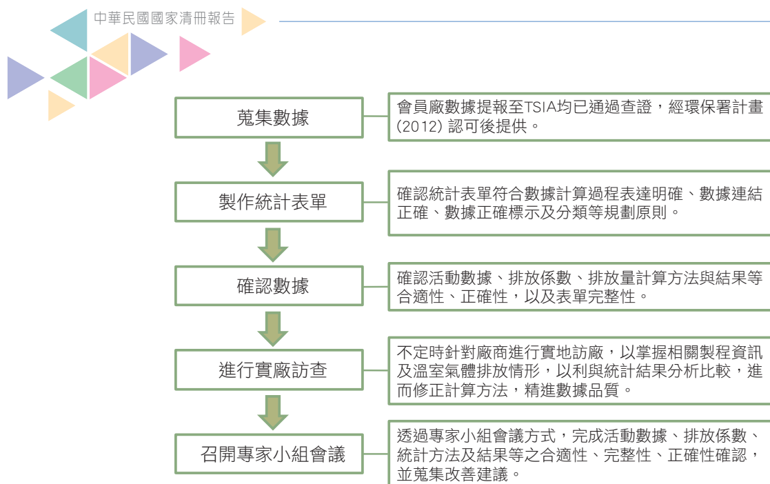
圖 4.6.5 TFT 平面顯示器排放統計 QA/QC 流程
