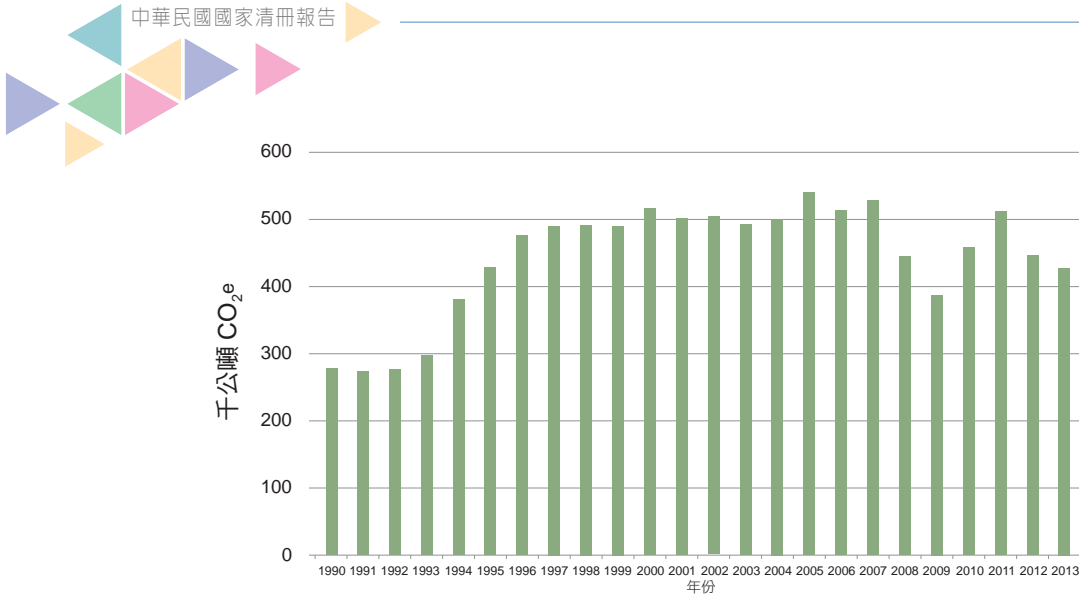
圖 4.3.13 臺灣 1990 至 2013 年碳煙生產排放量趨勢
