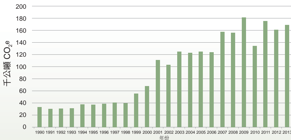
圖 4.3.11 臺灣 1990 至 2013 年環氧乙烷生產排放量趨勢
