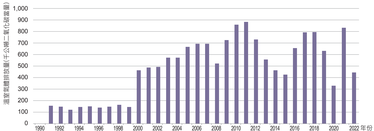
圖 4.3.3 1990 年至 2022 年己內醯胺生產製程排放量趨勢
