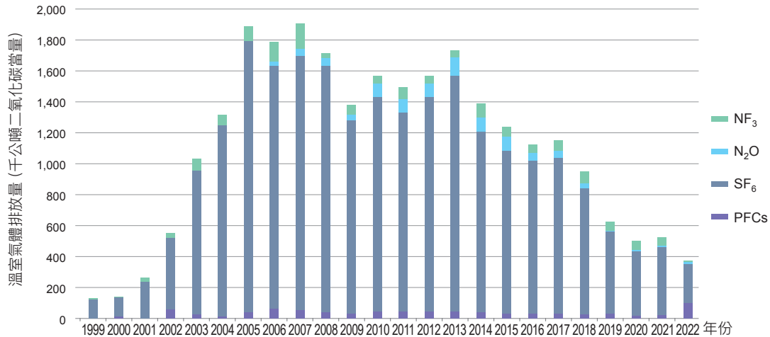
圖 4.6.4 1999 年至 2022 年 TFT 平面顯示器製程排放量趨勢
