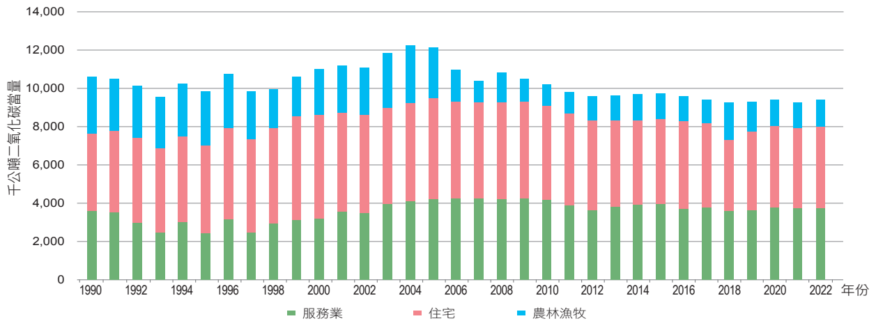
圖 3.2.26 1990 年至 2022 年服務業、住宅、農林漁牧燃料燃燒二氧化碳排放量趨勢
