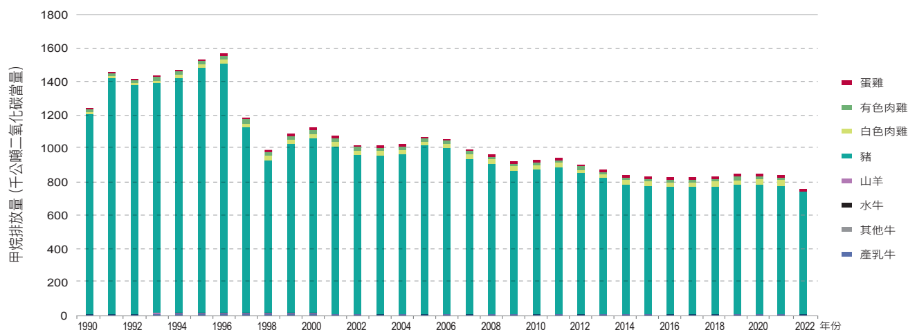
圖 5.3.1 1990 年至 2022 年畜禽糞尿處理之甲烷排放量
