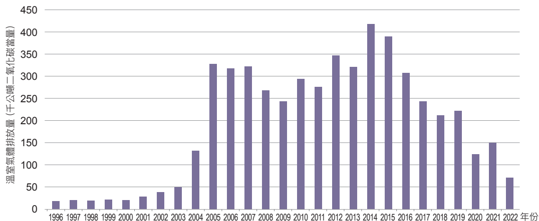
圖 4.3.10 1996 年至 2022 年環氧乙烷生產製程排放量趨勢
