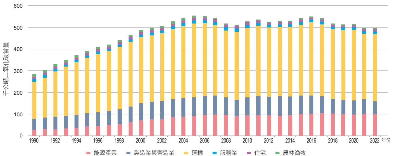
圖 3.2.3 1990 年至 2022 年能源部門燃料燃燒甲烷排放量趨勢
