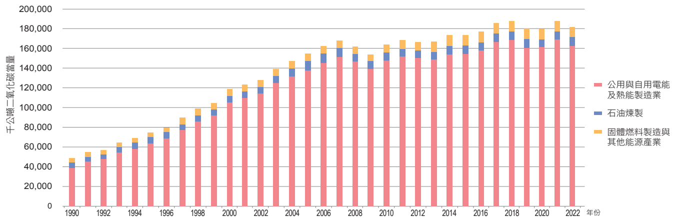
圖 3.2.8 1990 年至 2022 年能源產業燃料燃燒二氧化碳排放量趨勢
