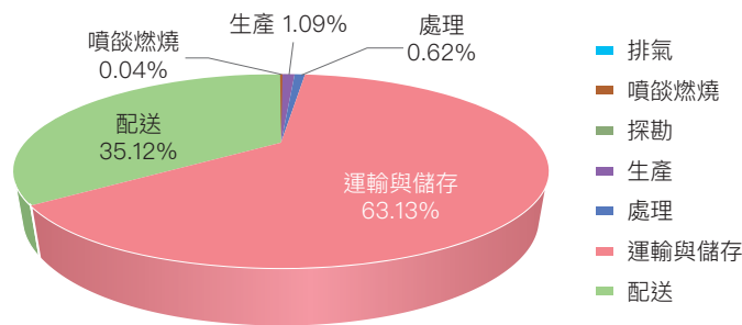
圖 3.3.8 2022 年天然氣逸散溫室氣體排放占比
