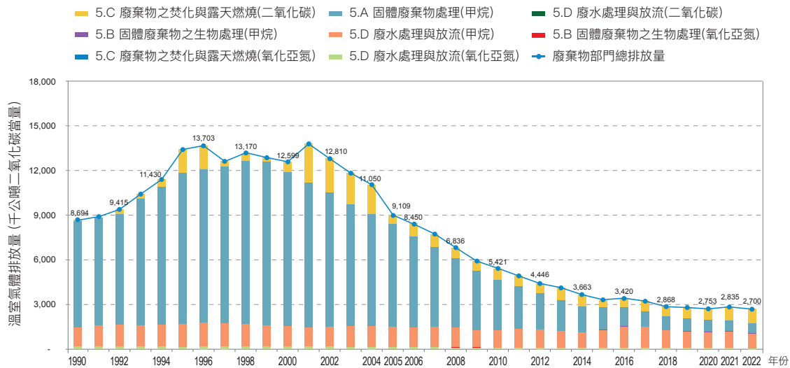
圖 2.3.6 1990 年至 2022 年廢棄物部門溫室氣體排放量趨勢
