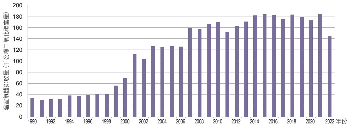
圖 4.3.8 1990 年至 2022 年乙烯生產製程排放量趨勢
