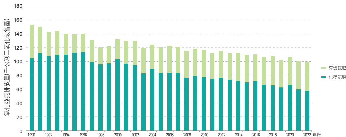
圖 5.5.3 1990 年至 2022 年農耕土壤間接氧化亞氮 – 揮散之排放量
