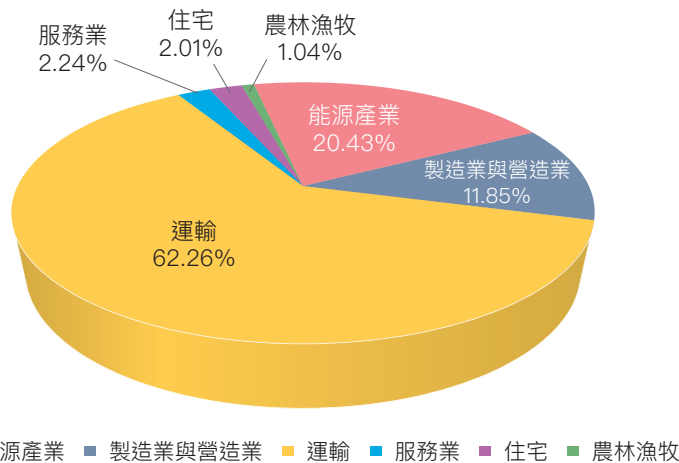
圖 3.2.4 2022 年能源部門燃料燃燒甲烷排放占比
