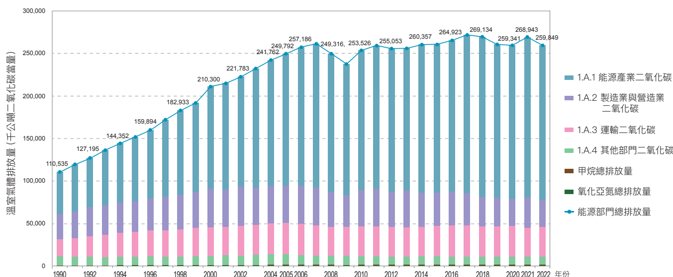
圖 2.3.2 1990 年至 2022 年能源部門溫室氣體排放量趨勢
