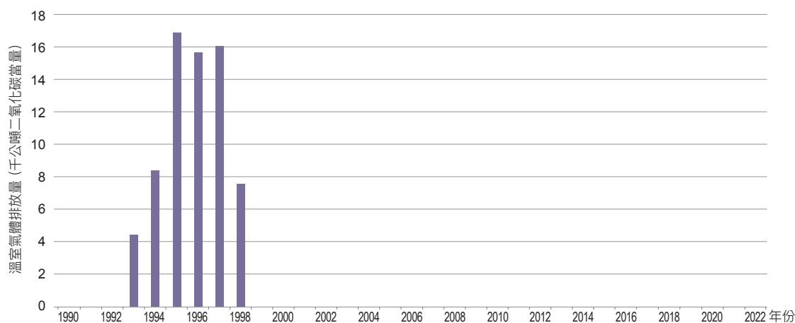
圖 4.3.7 1990 年至 2022 年甲醇生產製程排放量趨勢
