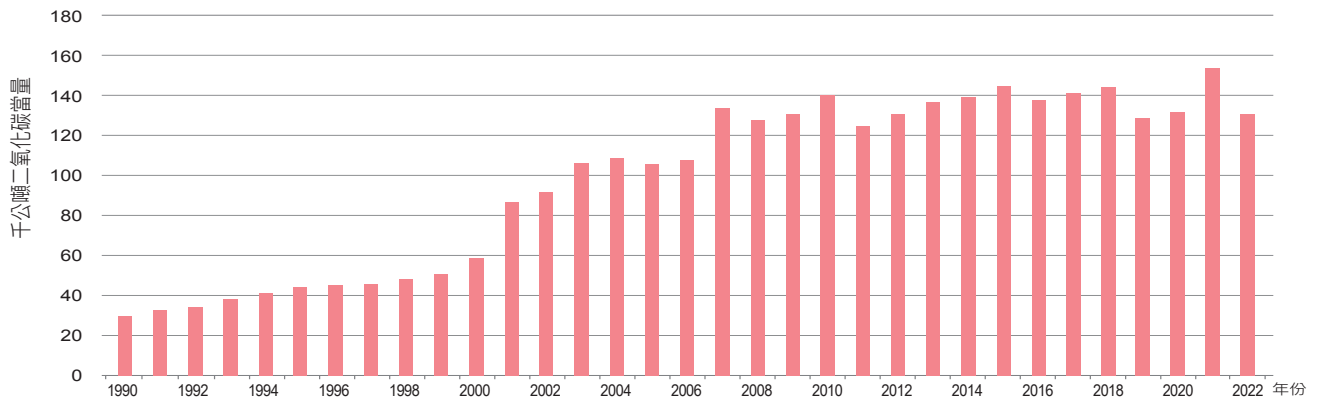
圖 3.2.40 1990 年至 2022 年非能源使用燃料燃燒氧化亞氮扣減量趨勢
