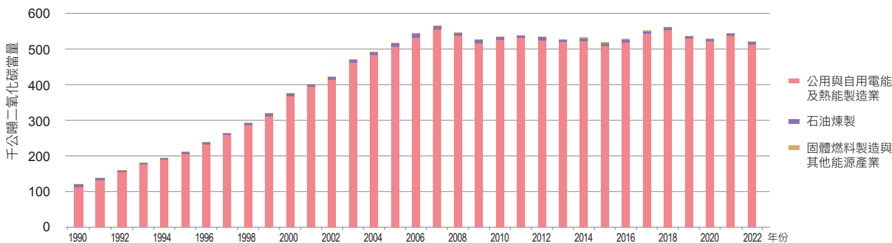
圖 3.2.12 1990 年至 2022 年能源產業燃料燃燒氧化亞氮排放量趨勢
