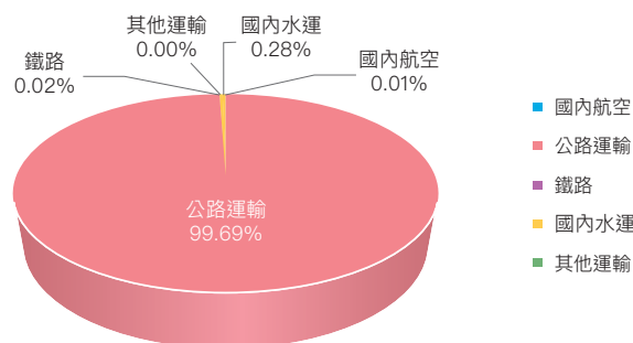
圖 3.2.23 2022 年運輸燃料燃燒甲烷排放占比
