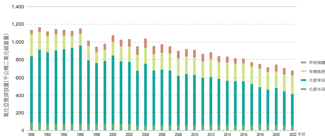
圖 5.5.2 1990 年至 2022 年農耕土壤直接氧化亞氮排放總量趨勢
