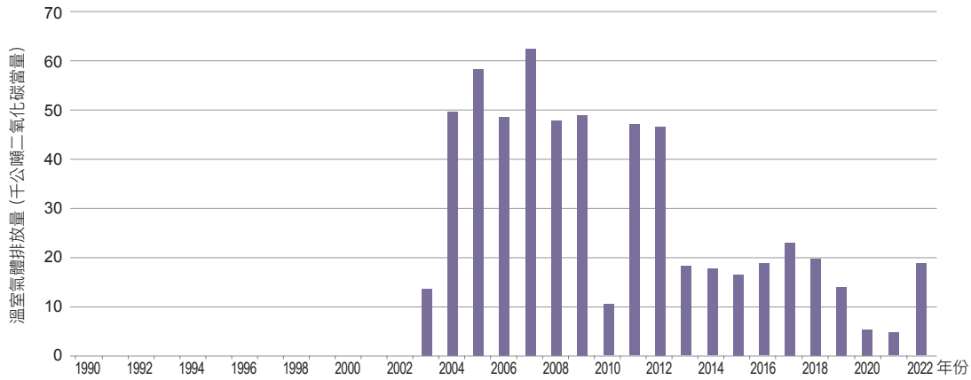
圖 4.4.8 1990 年至 2022 年鋅生產製程排放量趨勢
