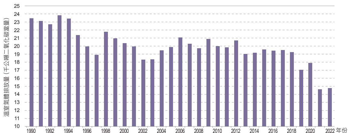
圖 4.9.2 1990 年至 2022 年啤酒生產製程排放量趨勢
