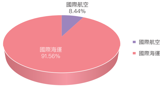
圖 3.2.35 2022 年國際運輸燃料燃燒甲烷排放占比
