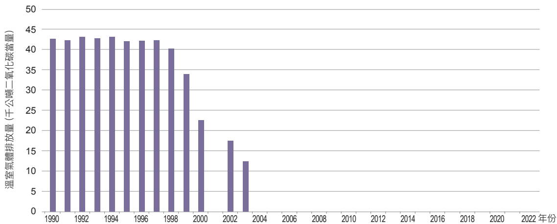
圖 4.3.4 1990 年至 2022 年碳化鈣生產製程排放量趨勢
