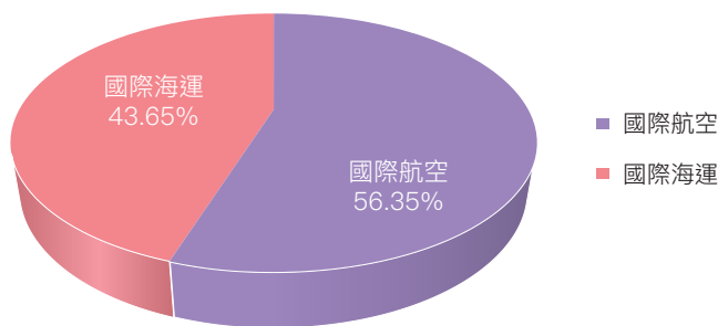
圖 3.2.37 2022 年國際運輸燃料燃燒氧化亞氮排放占比
