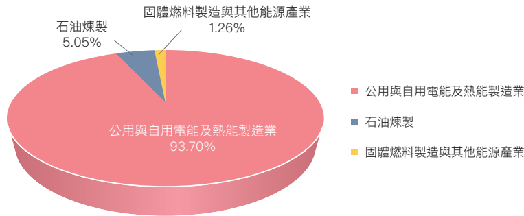
圖 3.2.11 2022 年能源產業燃料燃燒甲烷排放占比
