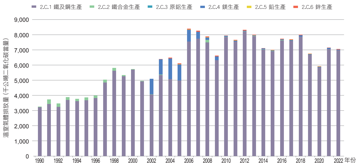
圖 4.4.1 1990 年至 2022 年金屬工業排放量趨勢
