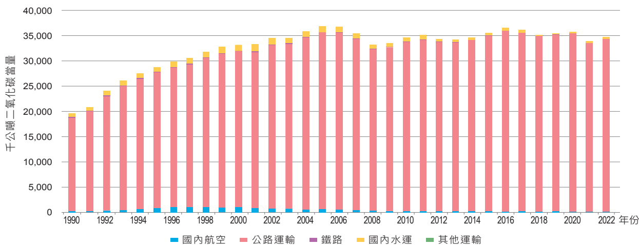
圖 3.2.20 1990 年至 2022 年運輸燃料燃燒二氧化碳排放量趨勢
