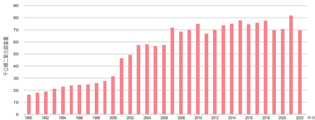
圖 3.2.39 1990 年至 2022 年非能源使用燃料燃燒甲烷扣減量趨勢
