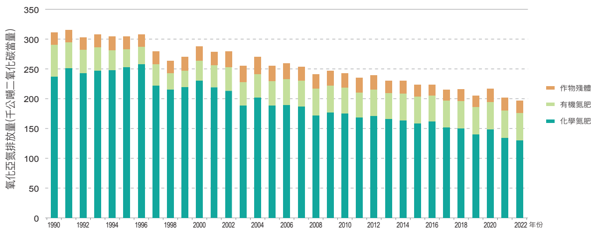
圖 5.5.4 1990 年至 2022 年農耕土壤間接氧化亞氮 – 淋洗 / 逕流之排放量
