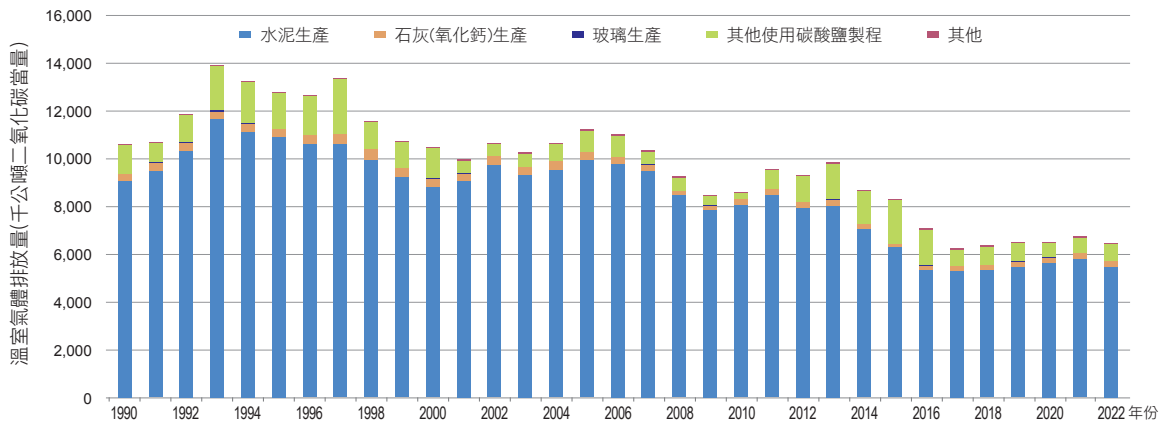
圖 4.2.1 1990 年至 2022 年礦業 (非金屬工業) 排放量趨勢
