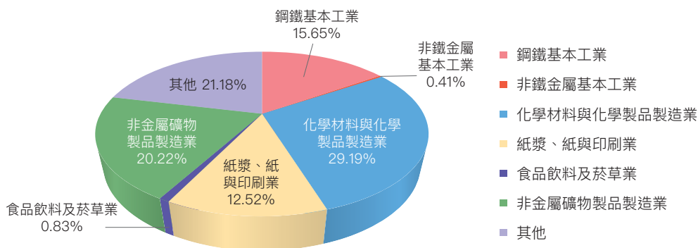
圖 3.2.19 2022 年製造業與營造業燃料燃燒氧化亞氮排放占比
