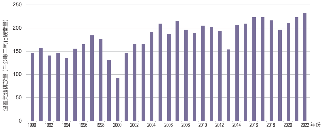
圖 4.3.2 1990 年至 2022 年硝酸生產製程排放量趨勢
