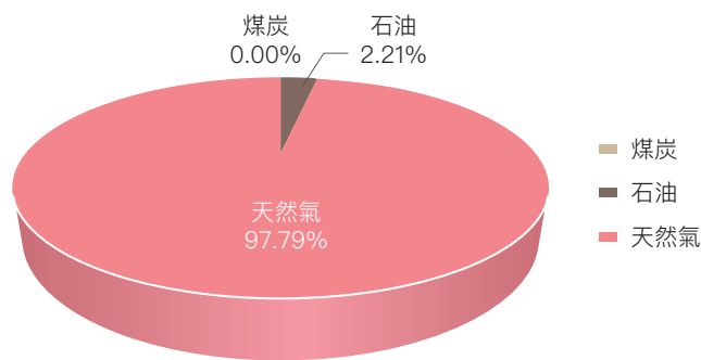
圖 3.3.2 2022 年能源部門燃料逸散溫室氣體排放占比
