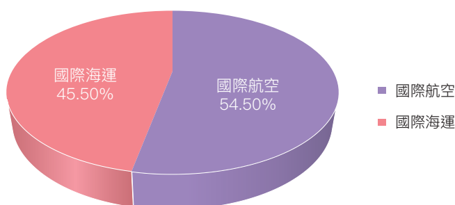
圖 3.2.33 2022 年國際運輸燃料燃燒二氧化碳排放占比
