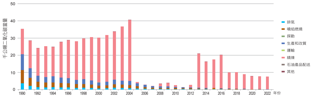
圖 3.3.5 1990 年至 2022 年石油逸散溫室氣體排放量趨勢
