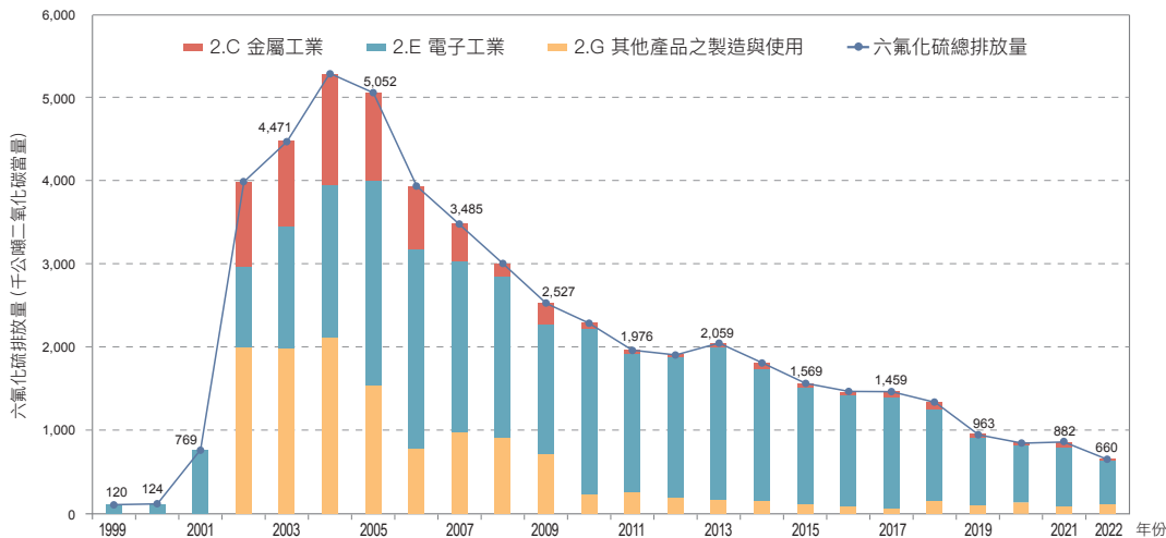
圖 2.2.6 1999 年至 2022 年六氟化硫排放量趨勢
