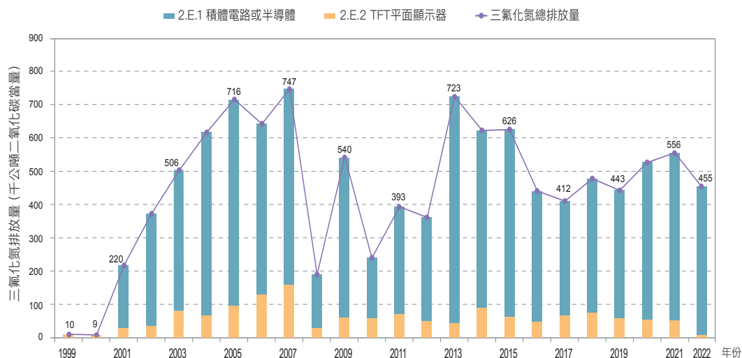
圖 2.2.7 1999 年至 2022 年三氟化氮排放量趨勢
