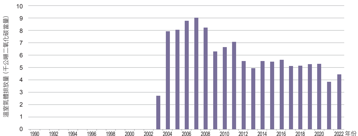
圖 4.4.7 1990 年至 2022 年鉛生產製程排放量趨勢
