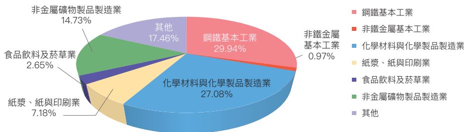
圖 3.2.15 2022 年製造業與營造業燃料燃燒二氧化碳排放占比
