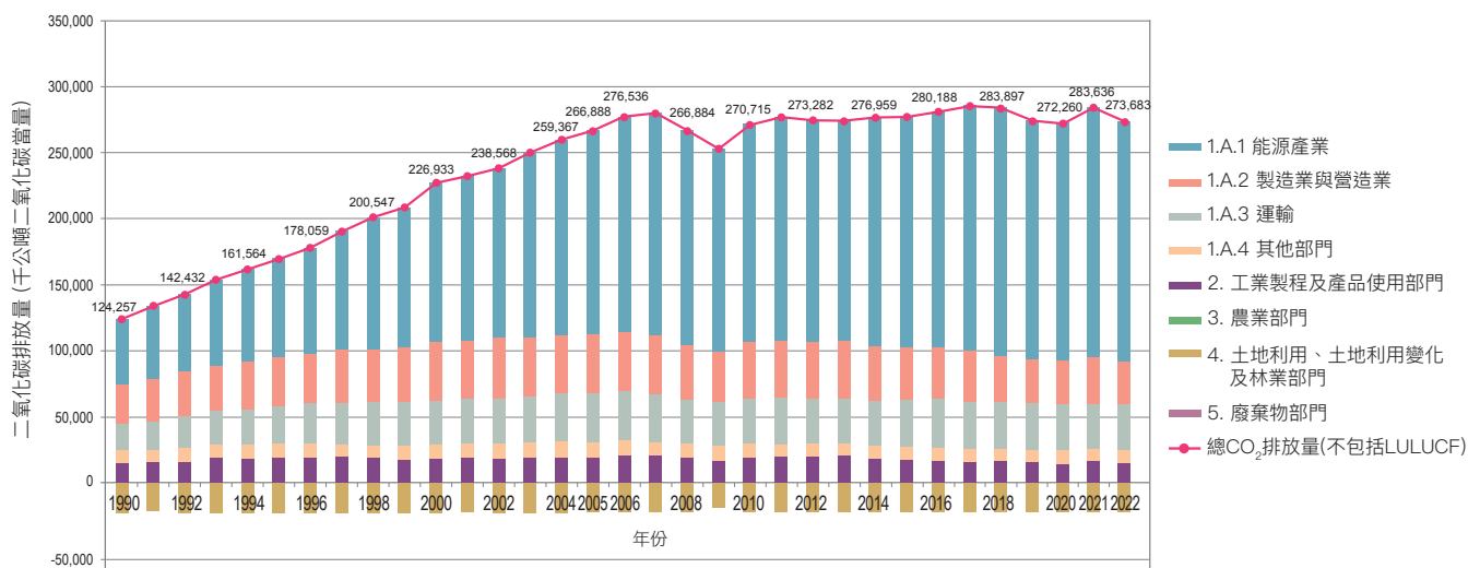
圖 2.2.1 1990 年至 2022 年二氧化碳排放量趨勢
