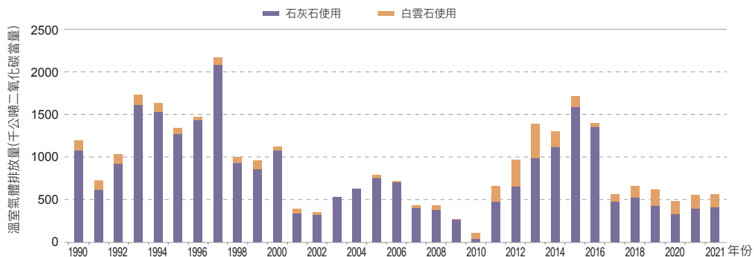
圖 4.2.7 1990 年至 2022 年石灰石與白雲石使用排放量趨勢
