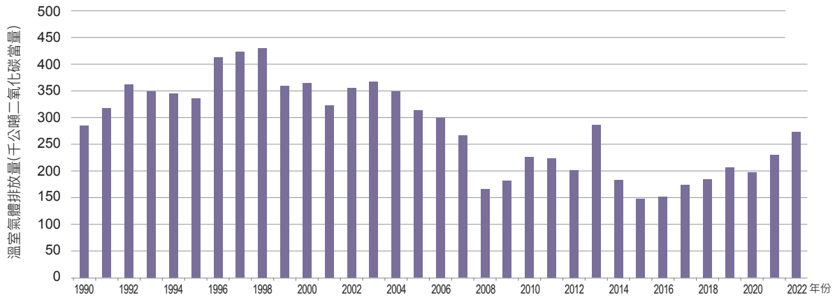
圖 4.2.4 1990 年至 2022 年石灰生產排放量趨勢
