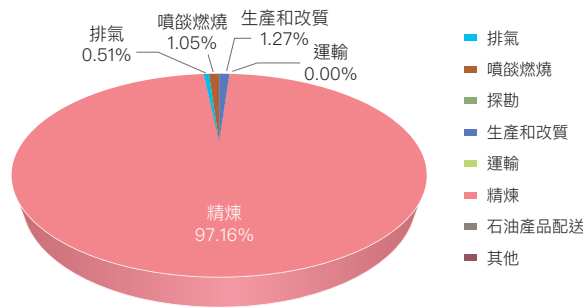
圖 3.3.6 2022 年石油逸散溫室氣體排放占比
