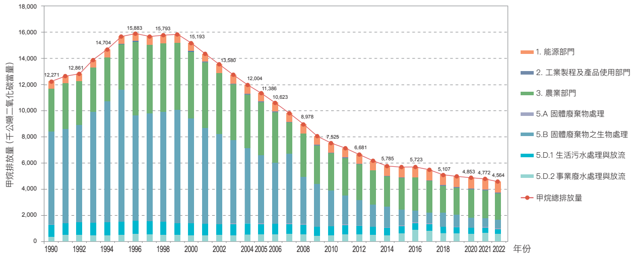
圖 2.2.2 1990 年至 2022 年甲烷排放量趨勢
