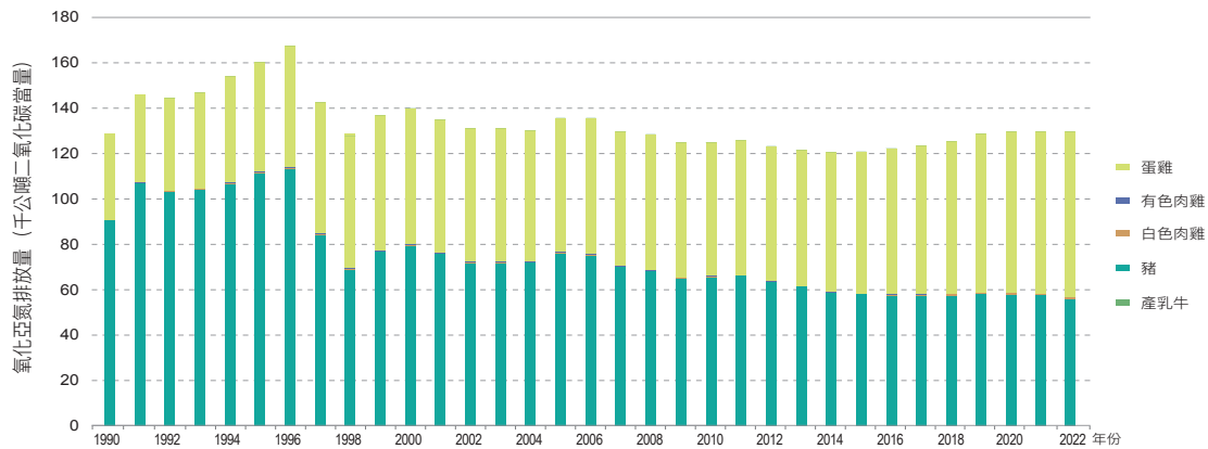
圖 5.3.2 1990 年至 2022 年畜禽糞尿處理之氧化亞氮排放量
