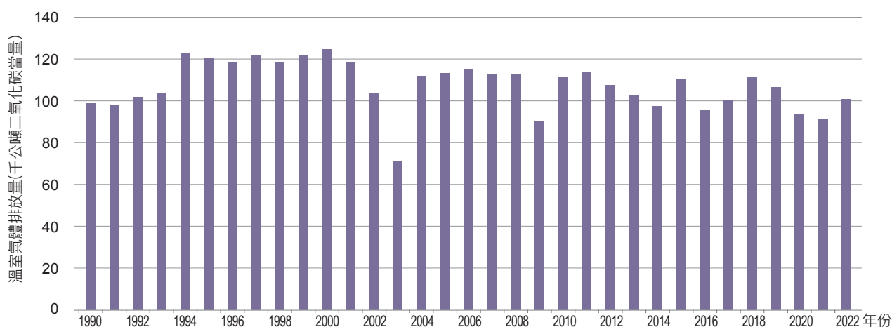
圖 4.2.6 1990 年至 2022 年純鹼使用排放量趨勢
