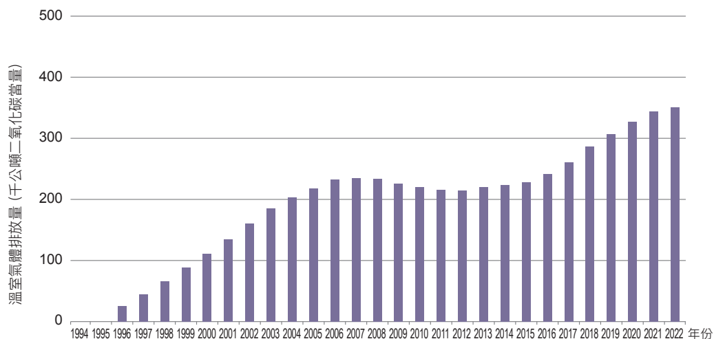
圖 4.7.3 1994 年至 2022 年車用空調之 HFCs 排放量趨勢
