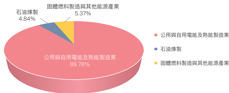
圖 3.2.9 2022 年能源產業燃料燃燒二氧化碳排放占比
