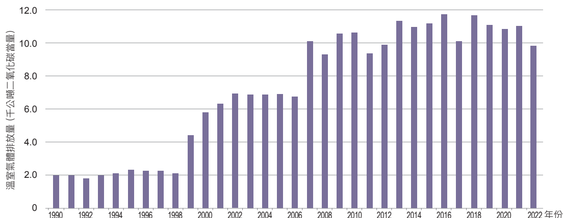
圖 4.3.14 1990 年至 2022 年苯乙烯生產製程排放量趨勢
