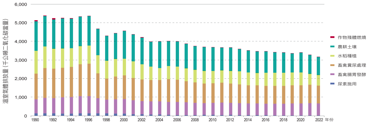
圖 5.1.1 1990 年至 2022 年農業部門排放量趨勢
