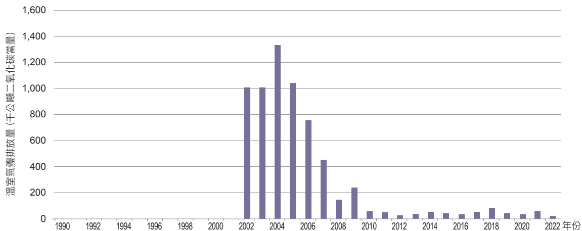
圖 4.4.5 1990 年至 2022 年鎂生產製程排放量趨勢
