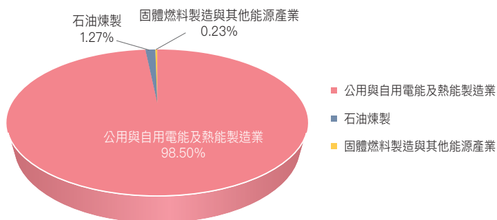
圖 3.2.13 2022 年能源產業燃料燃燒氧化亞氮排放占比
