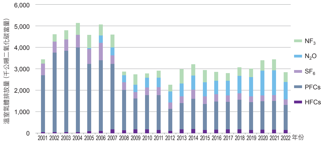
圖 4.6.2 2001 年至 2022 年積體電路或半導體製程排放量趨勢
