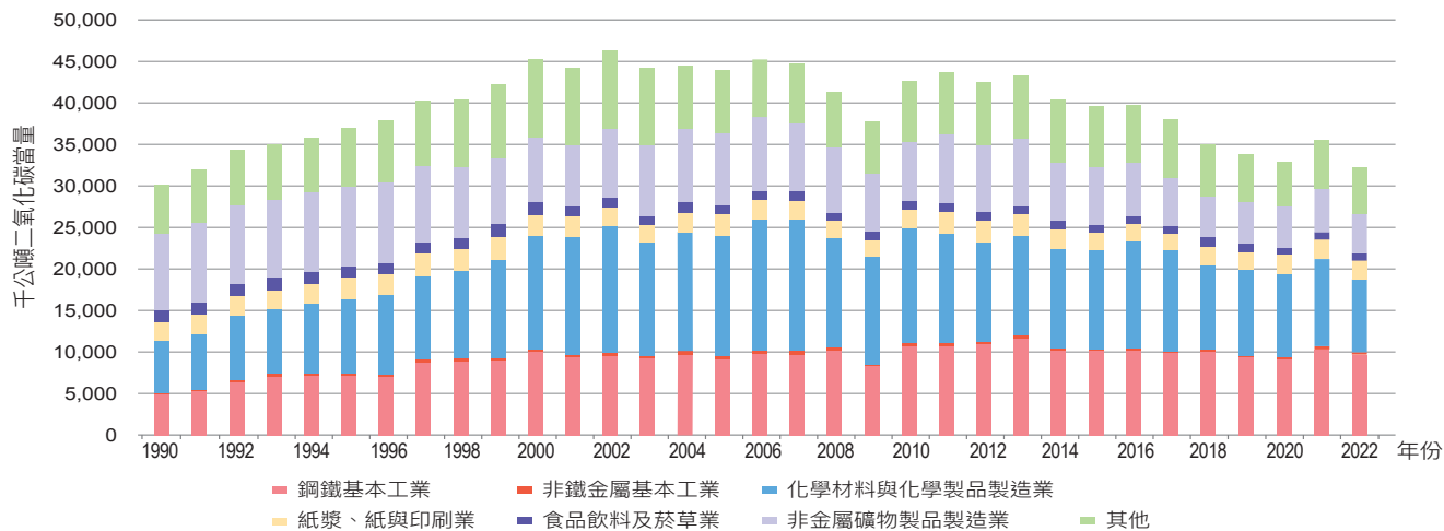
圖 3.2.14 1990 年至 2022 年製造業與營造業燃料燃燒二氧化碳排放量趨勢
