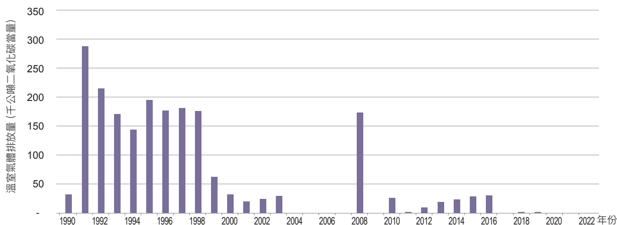
圖 4.4.4 1990 年至 2022 年鐵合金生產製程排放量趨勢
