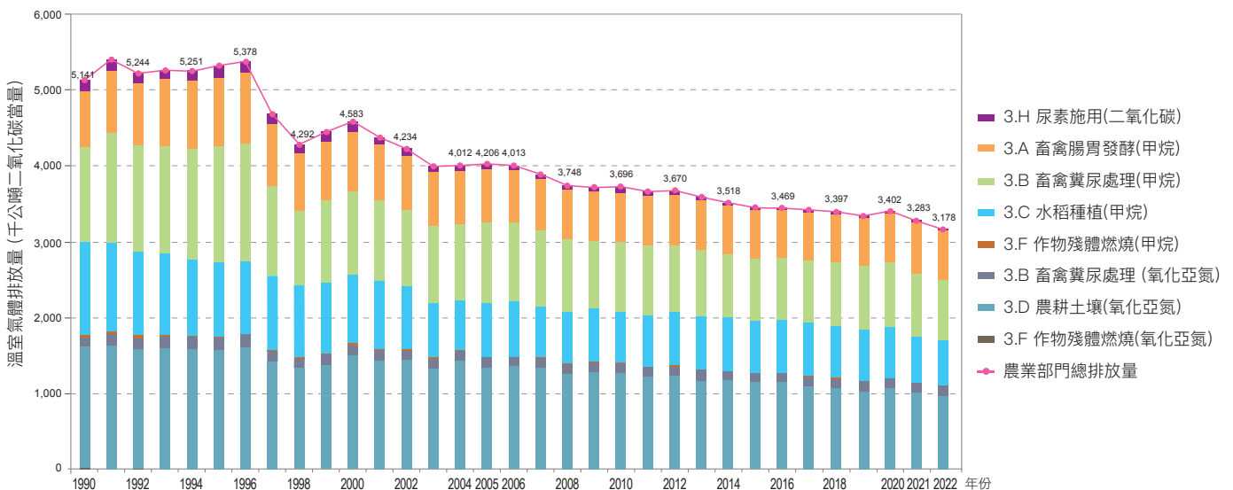
圖 2.3.4 1990 年至 2022 年農業部門溫室氣體排放量趨勢
