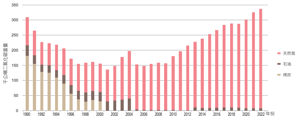
圖 3.3.1 1990 年至 2022 年能源部門燃料逸散溫室氣體排放量趨勢
