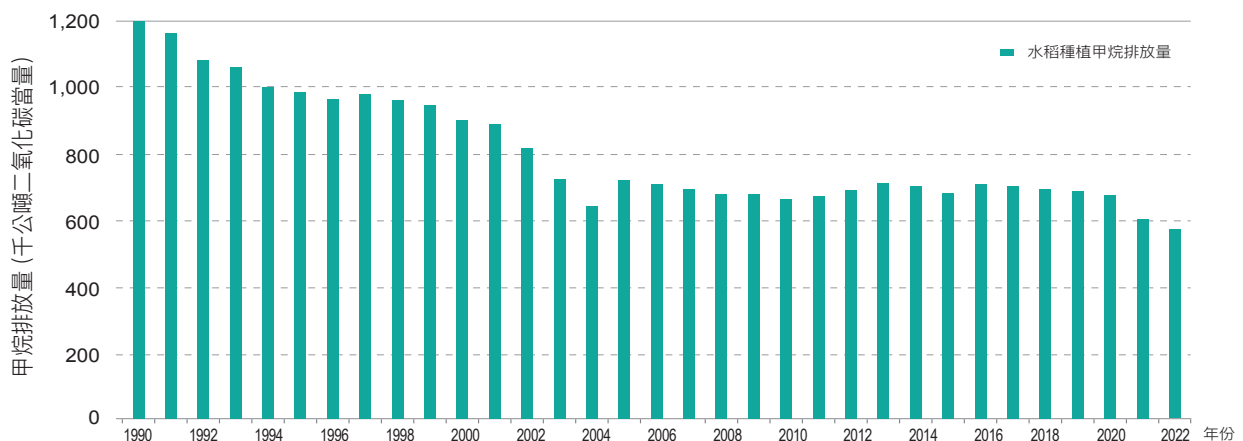
圖 5.4.1 1990 年至 2022 年水稻種植甲烷排放量
