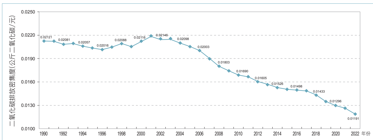
圖 2.1.3 1990 年至 2022 年二氧化碳排放密集度趨勢
