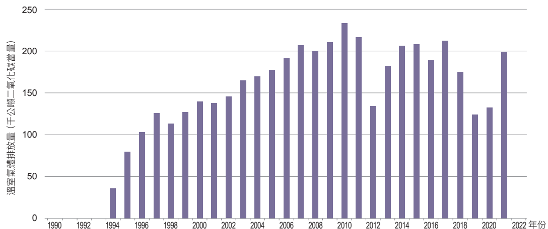
圖 4.3.5 1990 年至 2022 年二氧化鈦生產製程排放量趨勢
