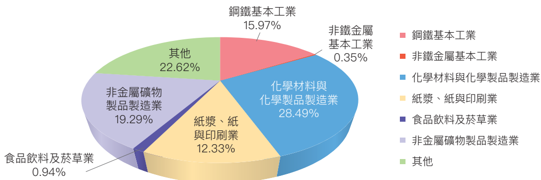
圖 3.2.17 2022 年製造業與營造業燃料燃燒甲烷排放占比
