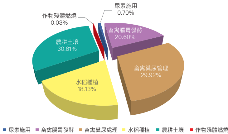
圖 5.1.2 2022 年農業部門溫室氣體各排放源占比
