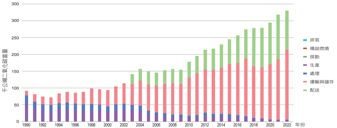
圖 3.3.7 1990 年至 2022 年天然氣逸散溫室氣體排放量趨勢
