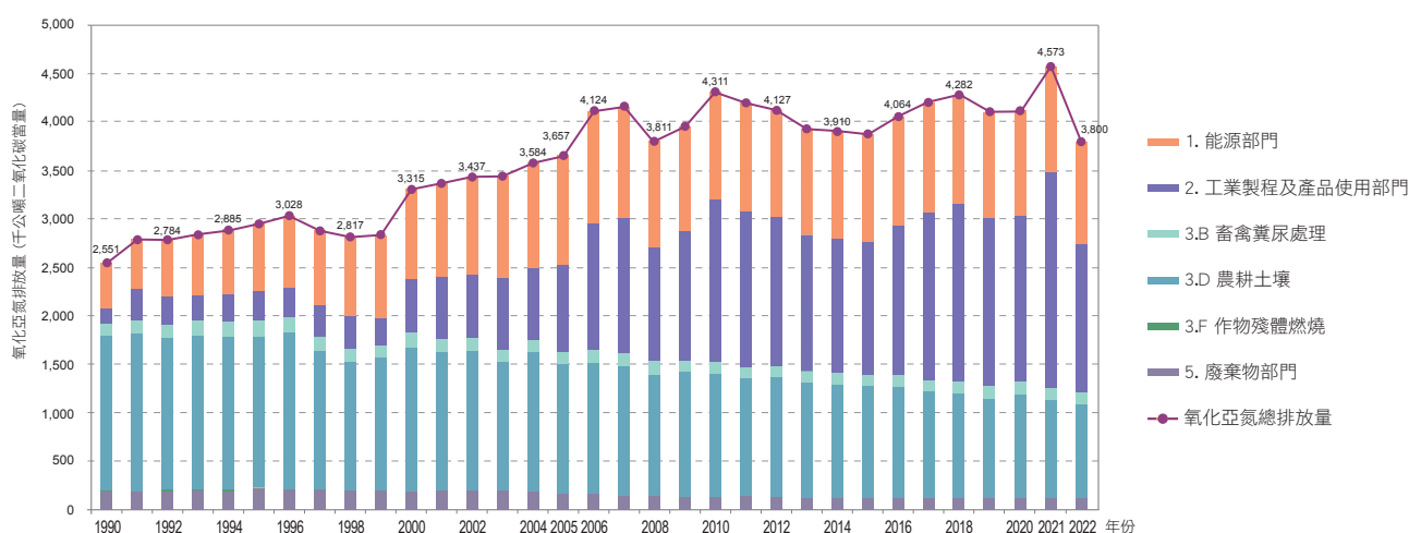
圖 2.2.3 1990 年至 2022 年氧化亞氮排放量趨勢
