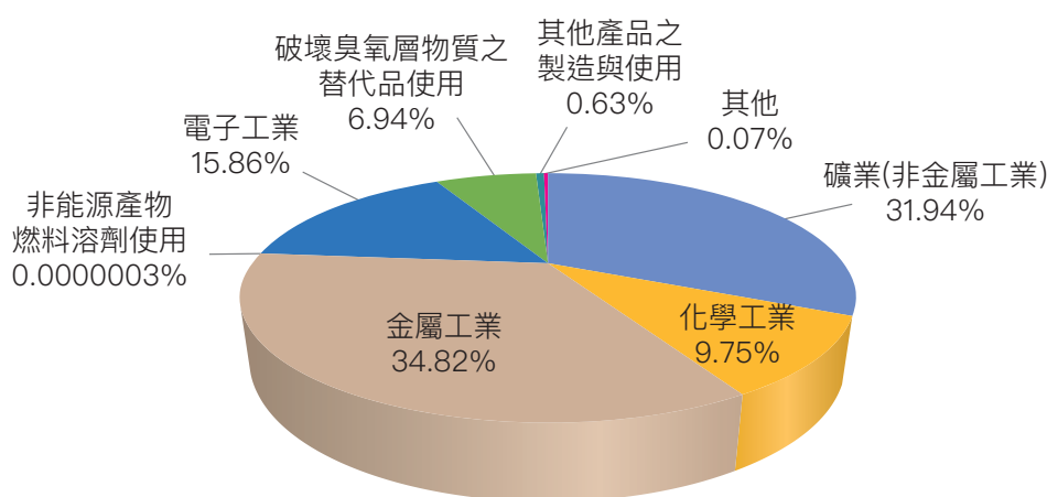
圖 4.1.2 2022 年工業製程及產品使用部門溫室氣體排放占比
