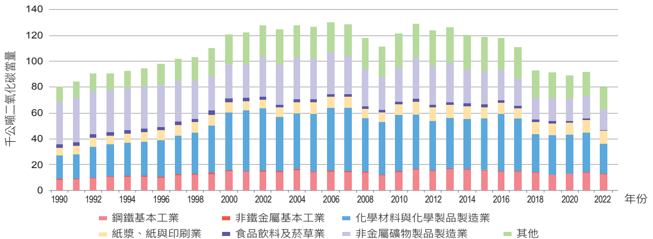
圖 3.2.18 1990 年至 2022 年製造業與營造業燃料燃燒氧化亞氮排放量趨勢
