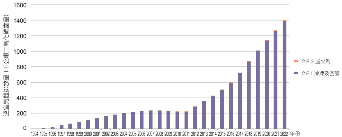
圖 4.7.1 1994 年至 2022 年破壞臭氧層物質之替代品使用排放量趨勢
