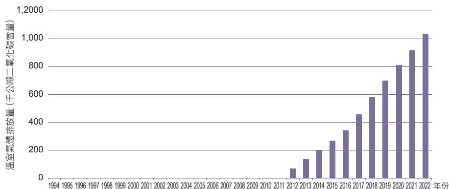
圖 4.7.4 1994 年至 2022 年固定式空調之 HFCs 排放量趨勢
