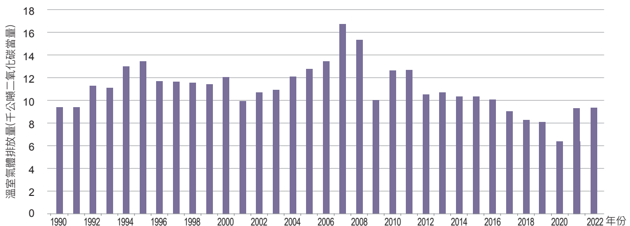
圖 4.2.5 1990 年至 2022 年玻璃生產排放量趨勢
