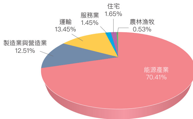
圖 3.2.2 2022 年能源部門燃料燃燒二氧化碳排放占比
