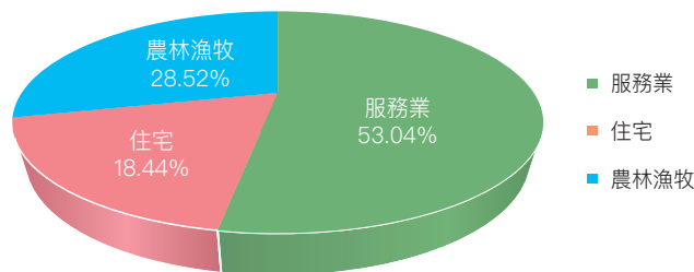
圖 3.2.31 2022 年服務業、住宅、農林漁牧燃料燃燒氧化亞氮排放占比
