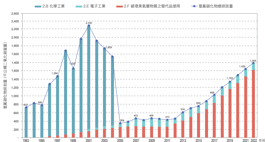
圖 2.2.4 1993 年至 2022 年氫氟碳化物排放量趨勢
