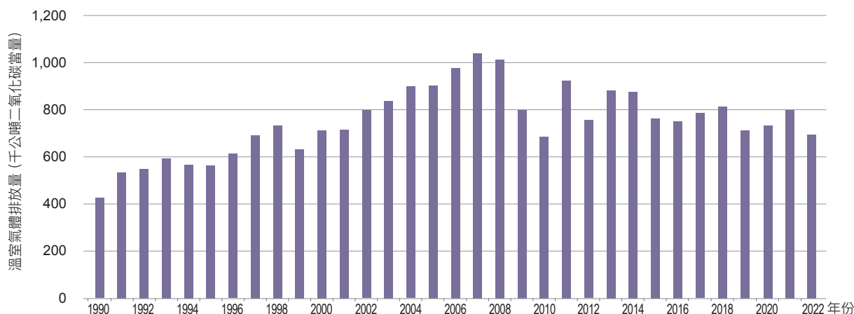
圖 4.4.3 1990 年至 2022 年電弧爐鋼胚生產製程排放量趨勢
