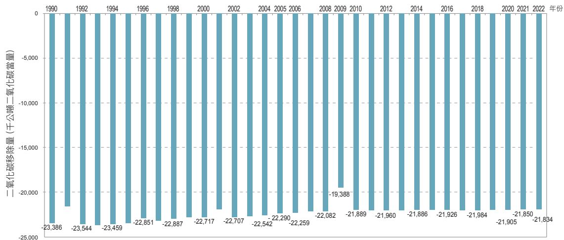
圖 2.3.5 1990 年至 2022 年土地利用、土地利用變化及林業部門碳移除量趨勢
