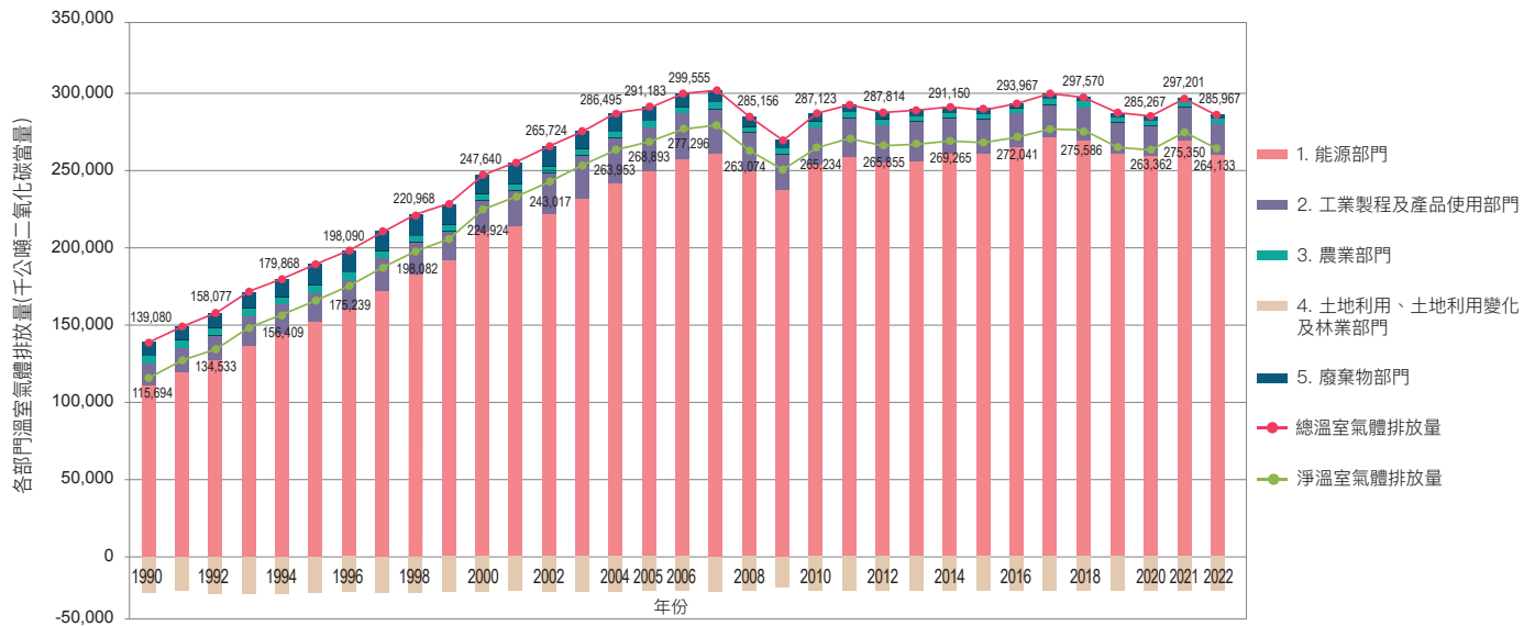
圖 2.3.1 1990 年至 2022 年各部門溫室氣體排放量趨勢
