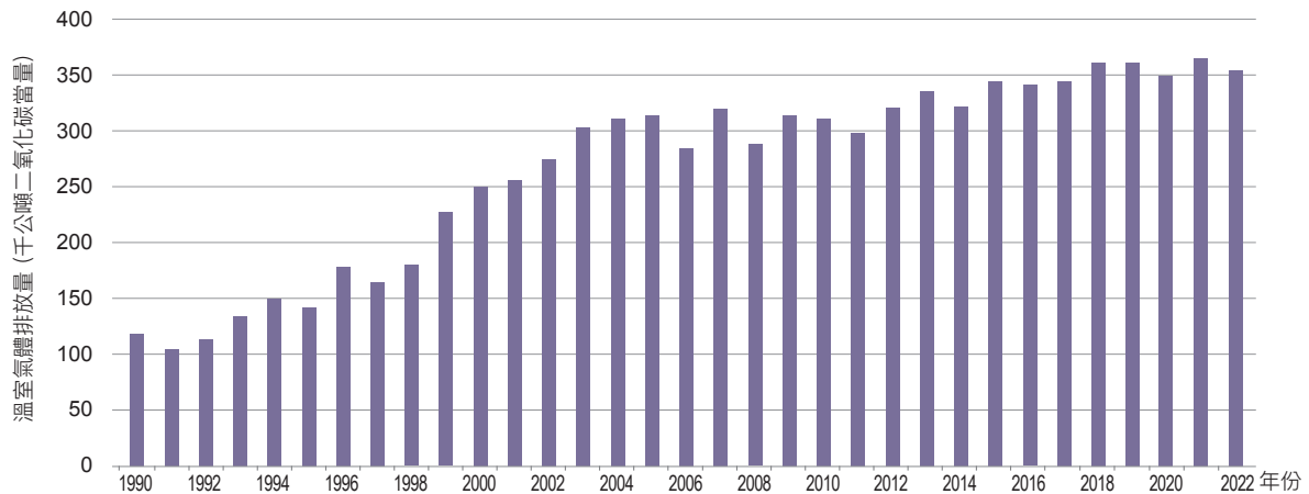
圖 4.3.9 1990 年至 2022 年氯乙烷生產製程排放量趨勢
