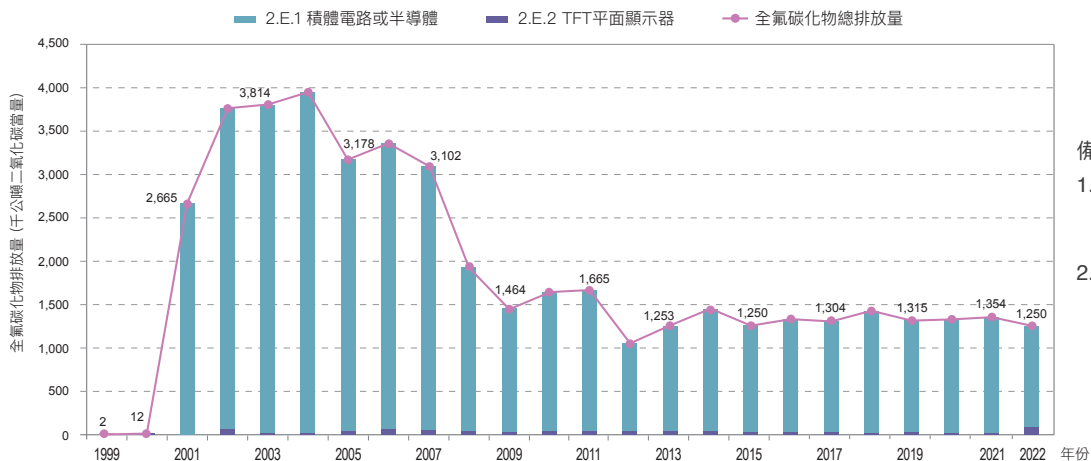
圖 2.2.5 1999 年至 2022 年全氟碳化物排放量趨勢
