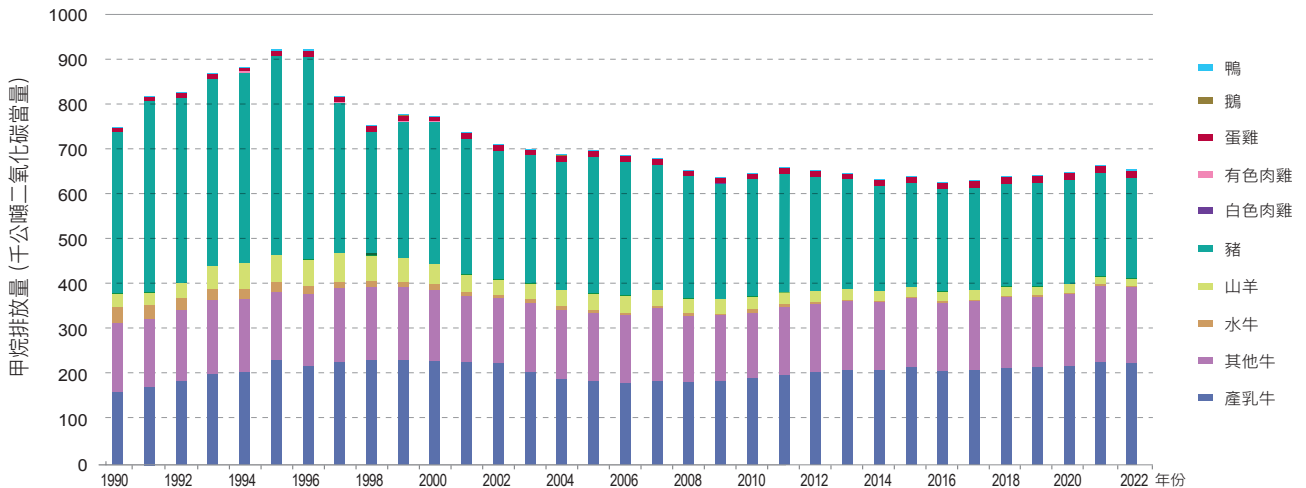
圖 5.2.1 1990 年至 2022 年畜禽腸胃發酵之甲烷排放量
